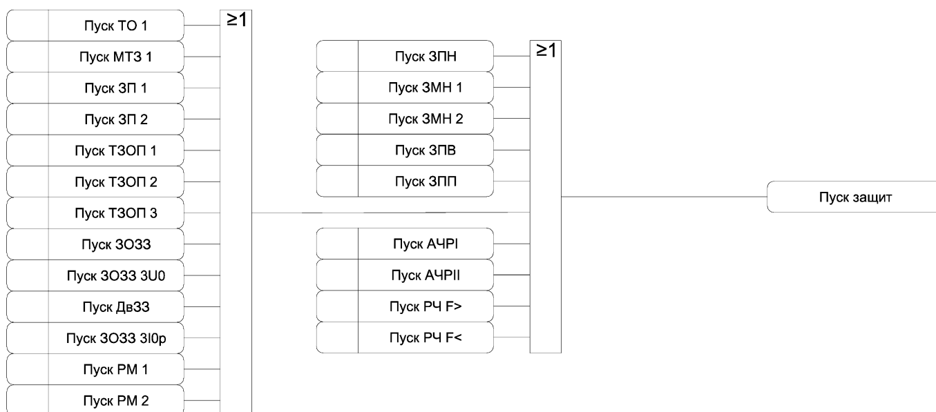
Рисунок 3.37 а) – Функциональная схема алгоритма формирования сигналов состояния защит
