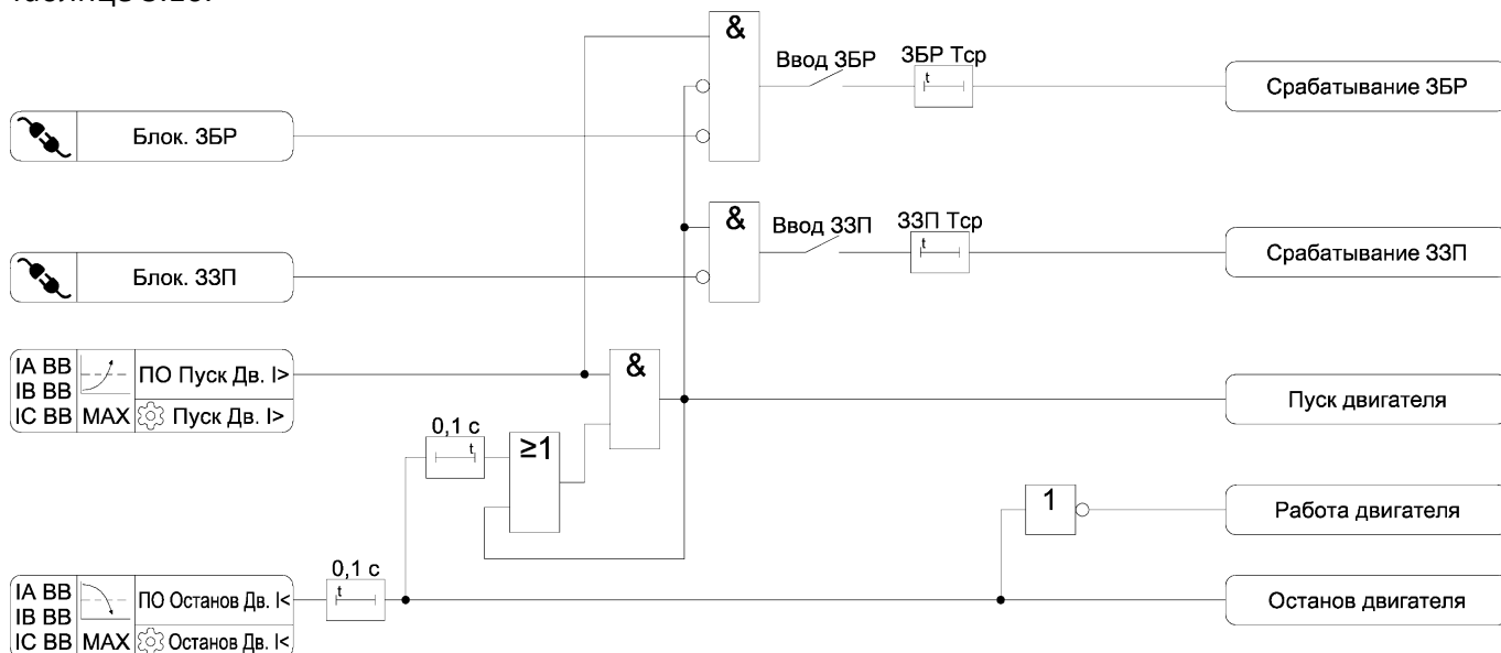
Рисунок 3.9 – Функциональная схема алгоритма 3ЗП и 3БР
