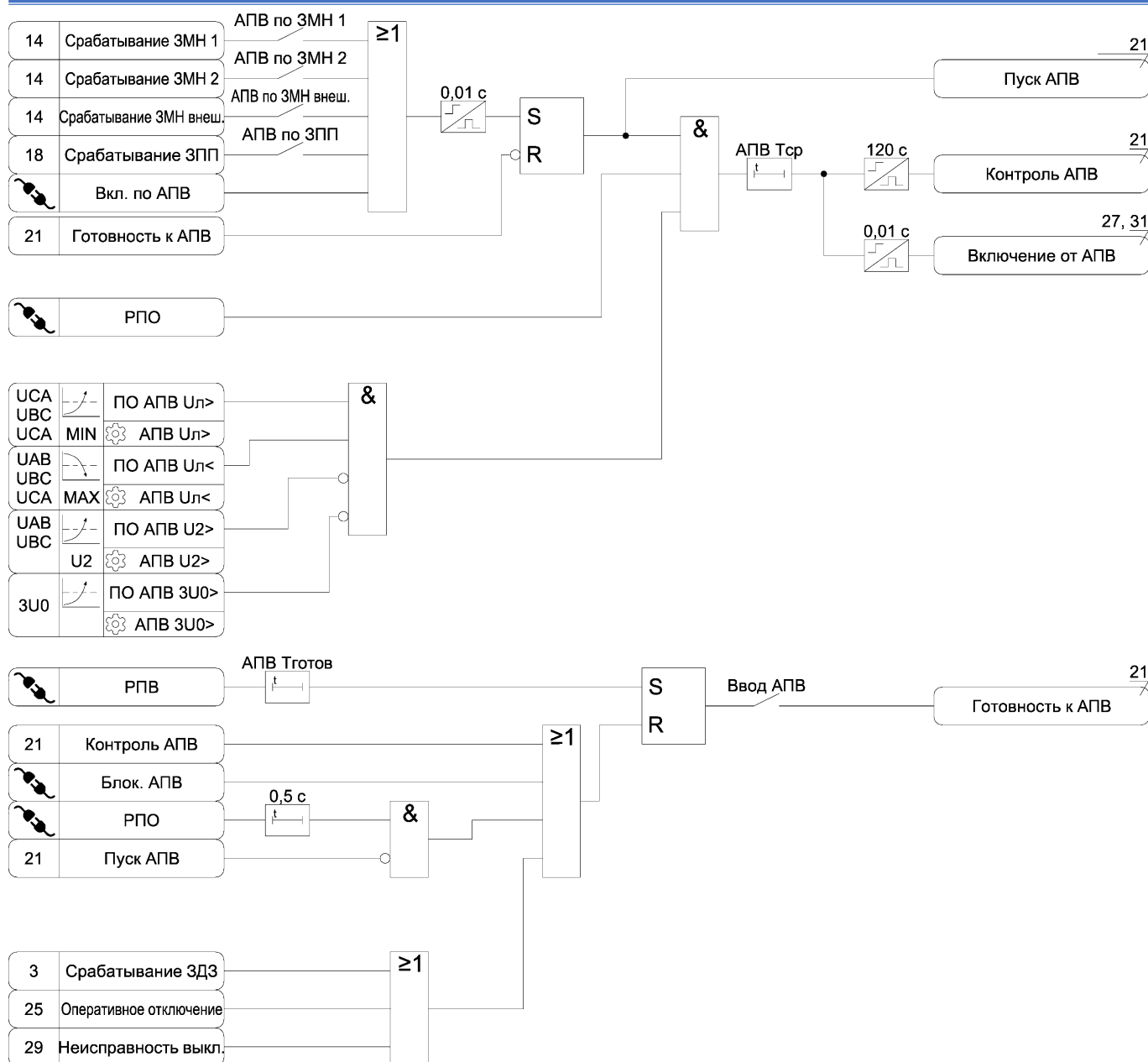
Рисунок А.21 – Функциональная схема алгоритма АПВ
