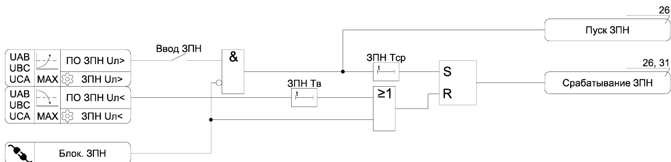
Рисунок А.13 – Функциональная схема алгоритма ЗПН
