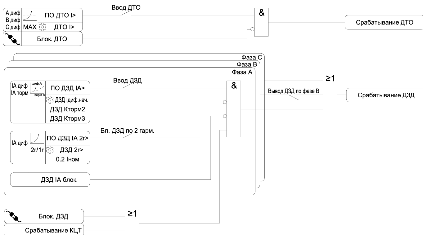
Рисунок 3.1 – Функциональная схема алгоритма ДЗД
