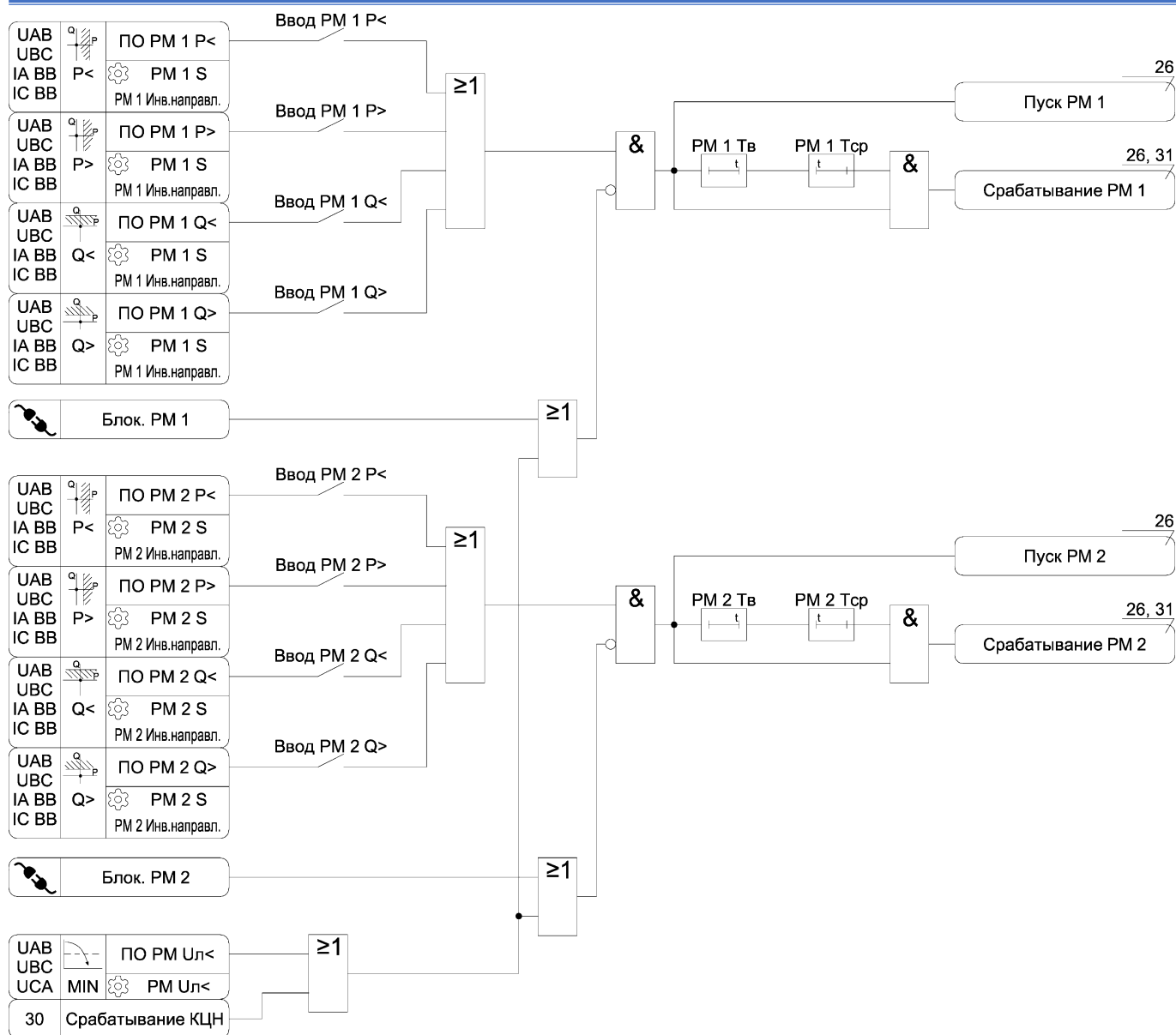
Рисунок А.12 – Функциональная схема алгоритма защиты по направлению мощности
