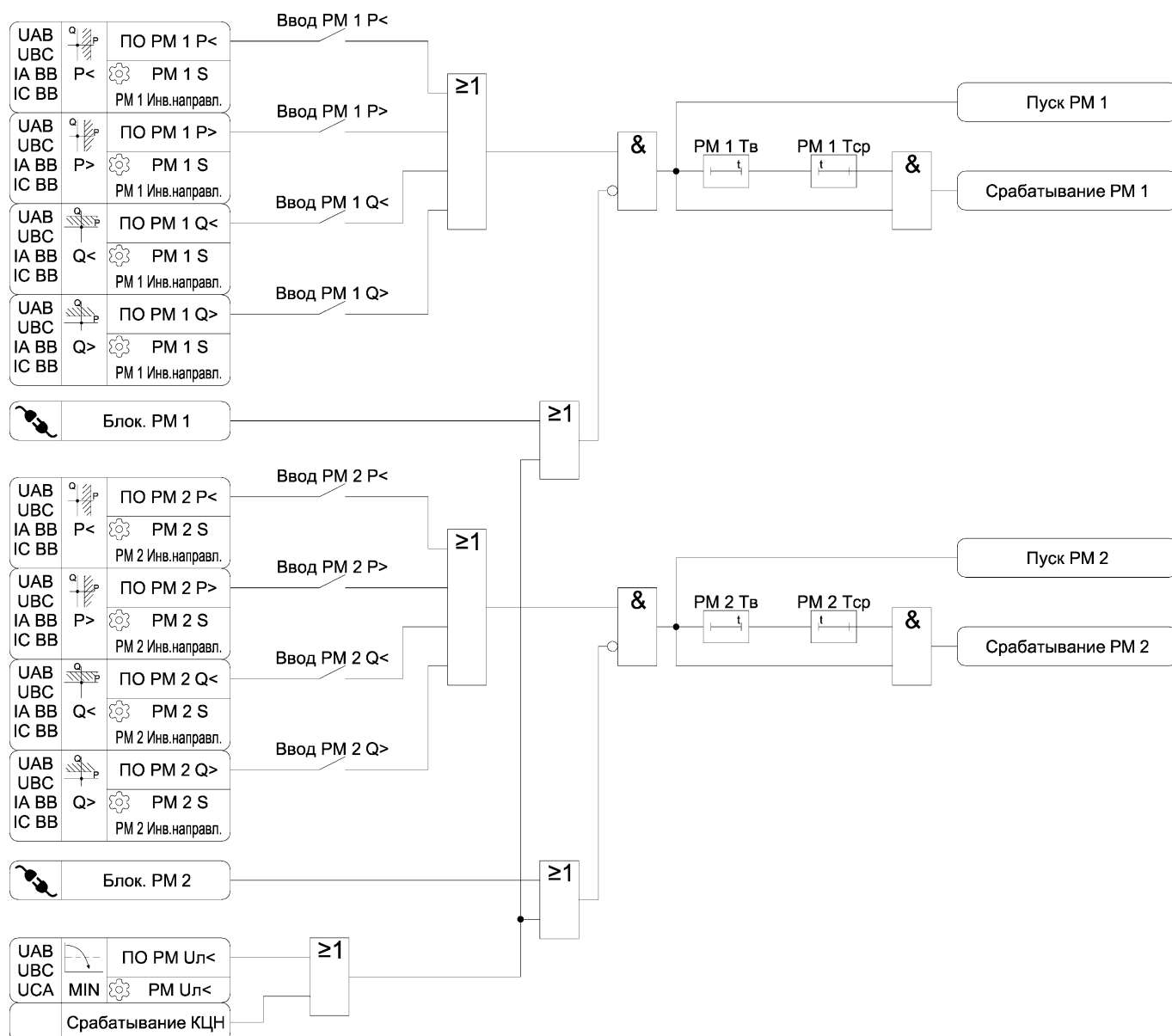
Рисунок 3.17 – Функциональная схема алгоритма защиты по направлению мощности
