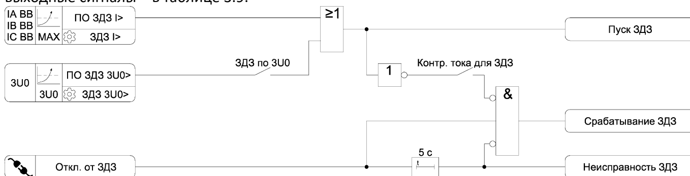
Рисунок 3.6 – Функциональная схема алгоритма ЗДЗ
