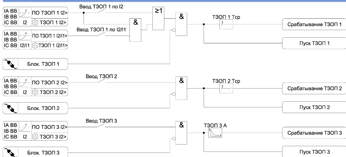
Рисунок 3.11 – Функциональная схема алгоритма ТЗОП
