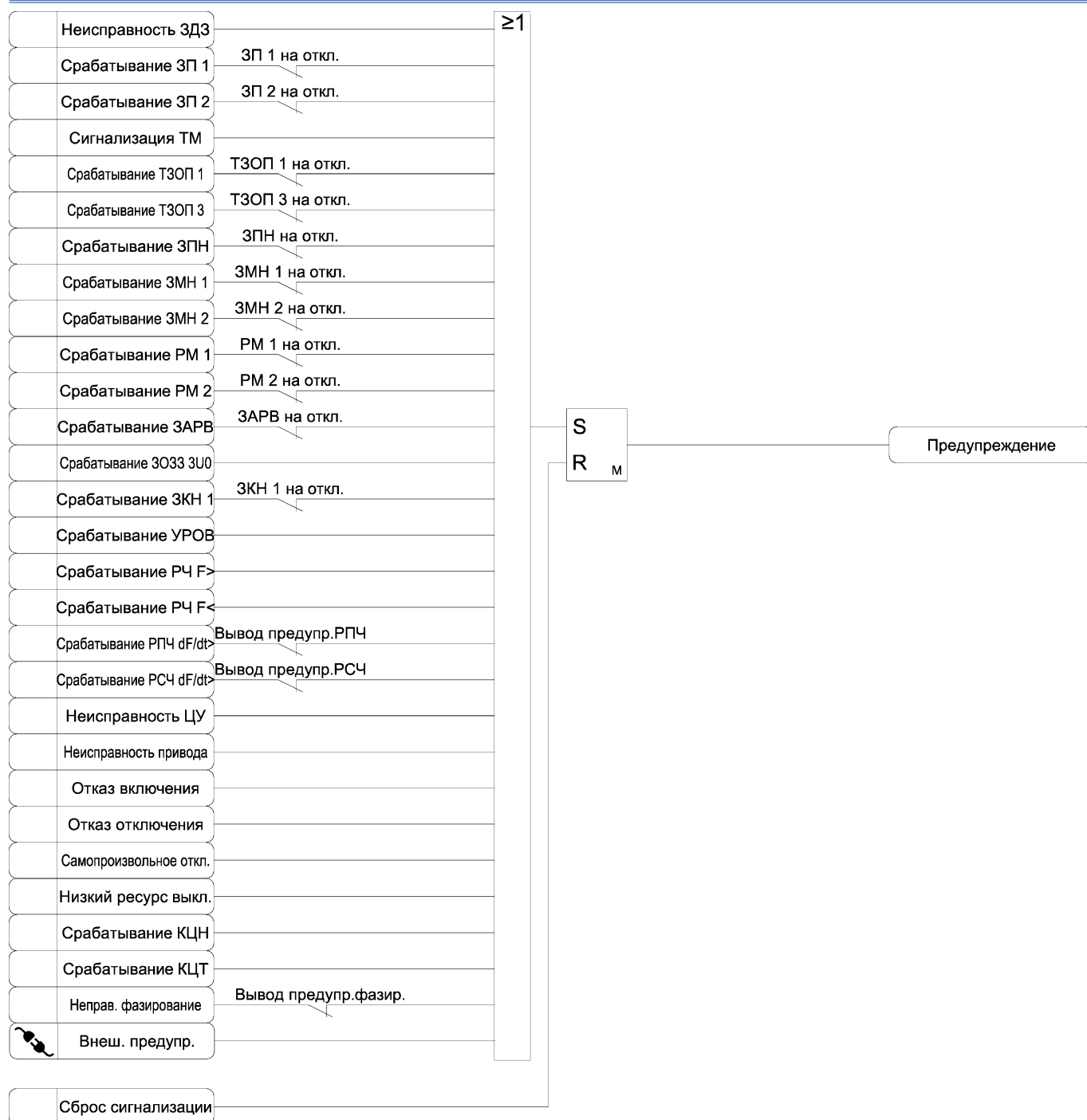
Рисунок 3.41 в) – Функциональная схема алгоритма сигнализации
