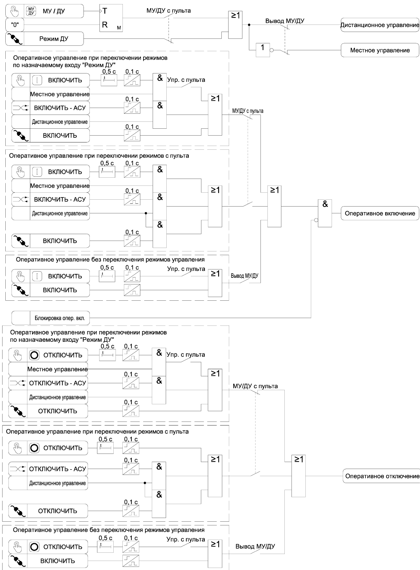
Рисунок 3.35 – Функциональная схема алгоритма оперативного управления выключателем
