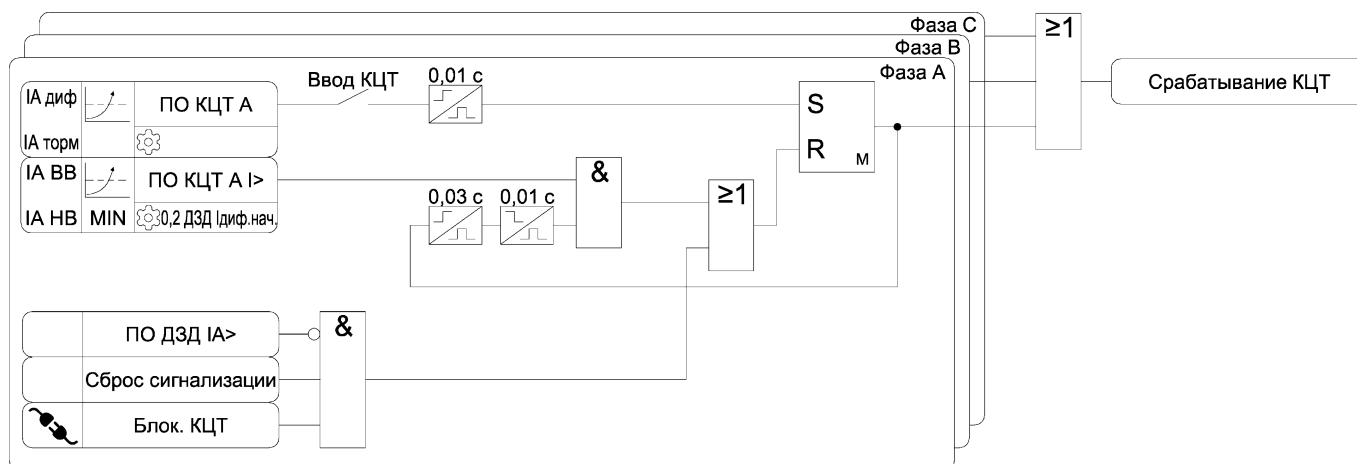
Рисунок 3.13 – Функциональная схема алгоритма КЦТ
