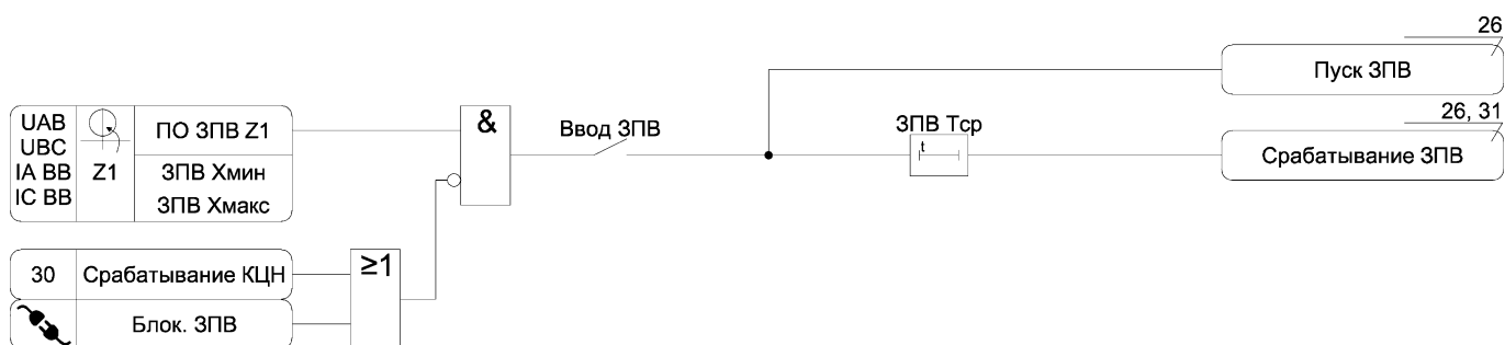
Рисунок А.15 – Функциональная схема алгоритма 3ПВ
