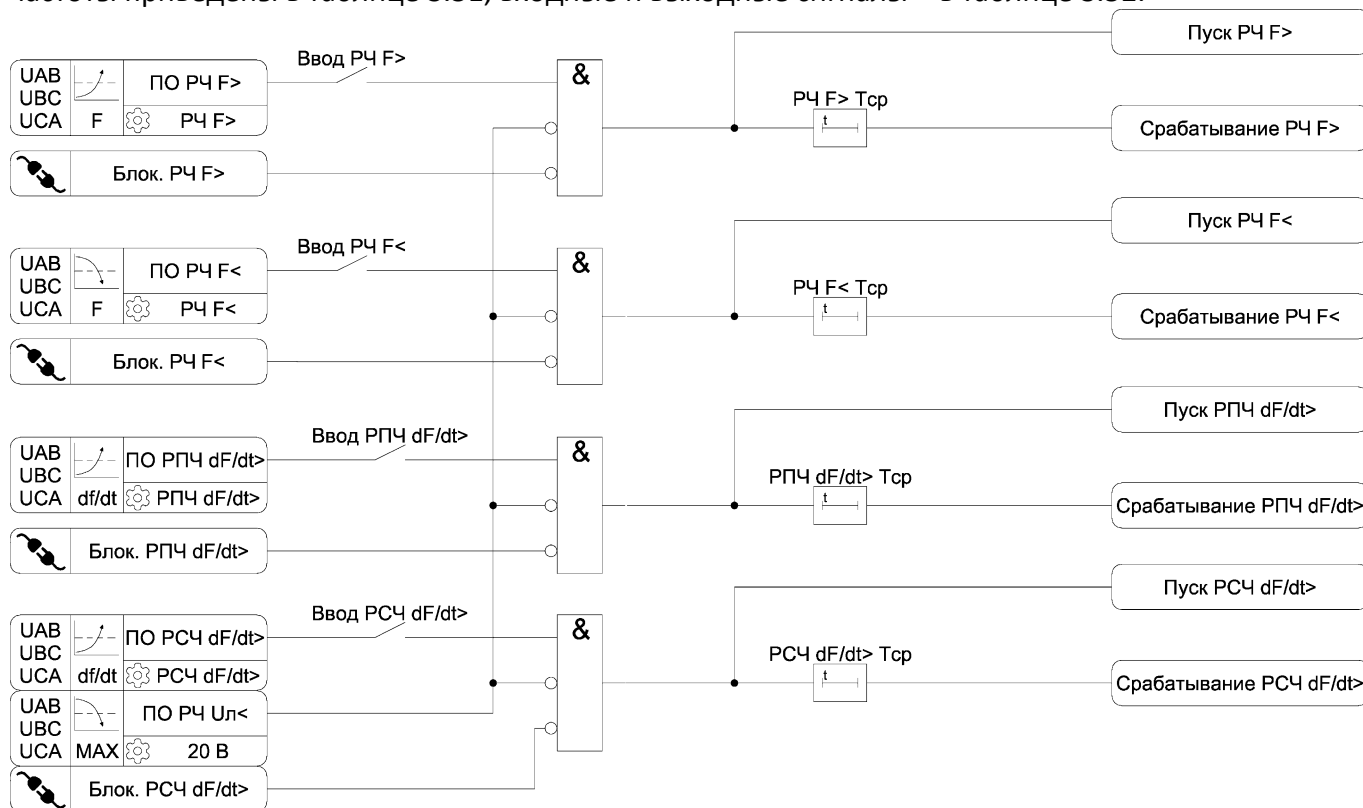
Рисунок 3.34 – Функциональные схемы алгоритмов защиты повышения и снижения частоты
