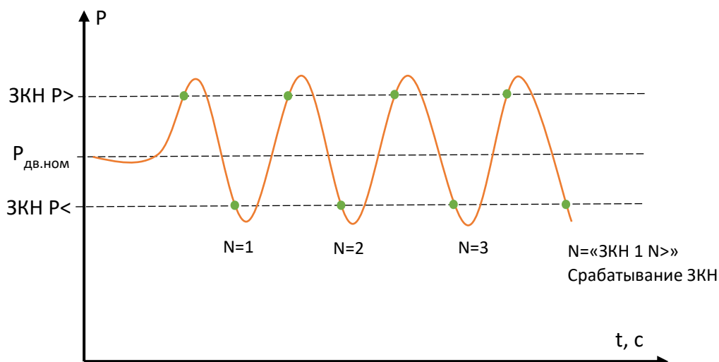
Рисунок 3.29 Временная диаграмма работы ЗКН
