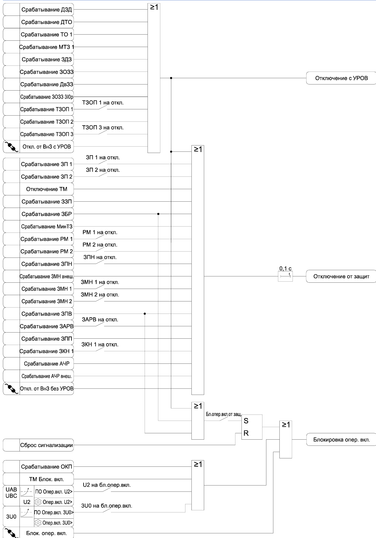
Рисунок 3.37 б) – Функциональная схема алгоритма формирования сигналов состояния защит
