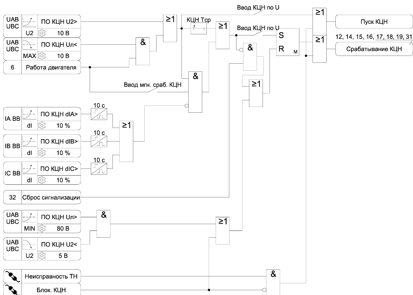
Рисунок А.30 – Функциональная схема алгоритма КЦН
