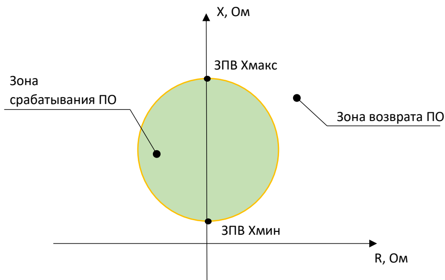
Рисунок 3.22 Характеристика срабатывания ЗПВ
