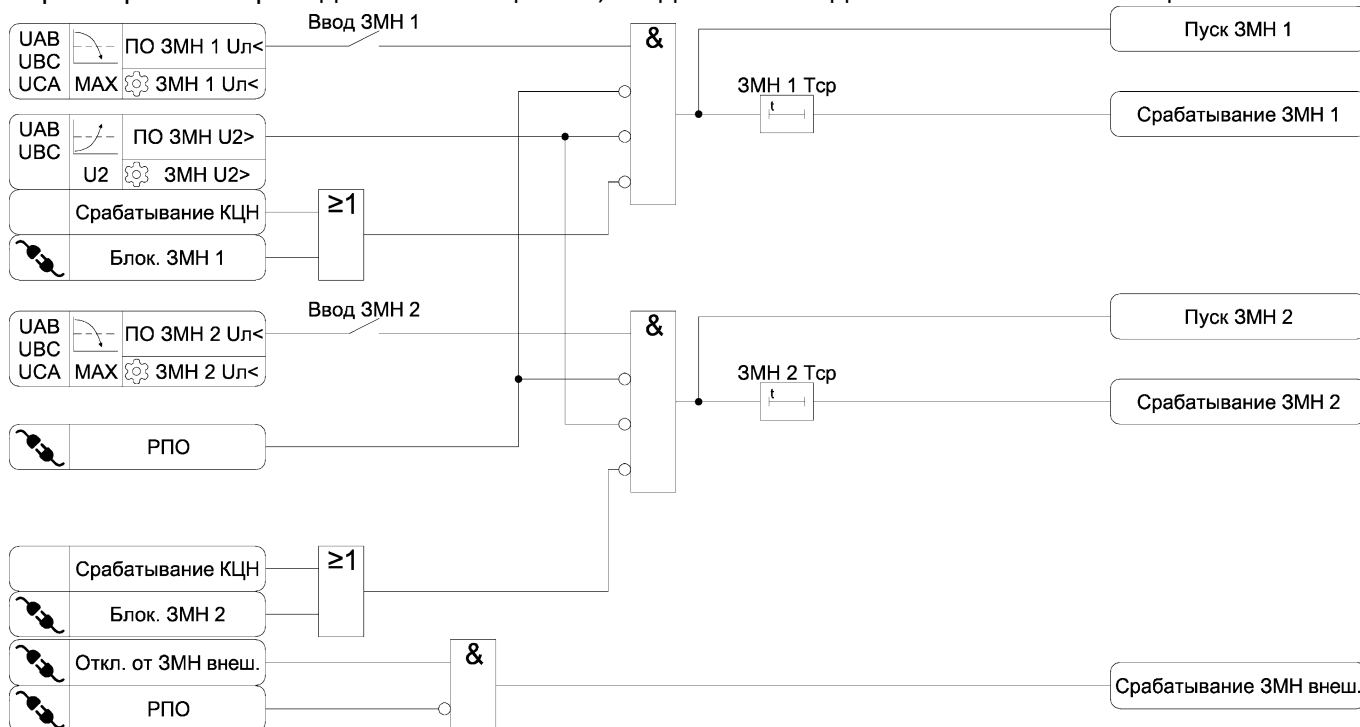
Рисунок 3.20 – Функциональная схема алгоритма ЗМН
