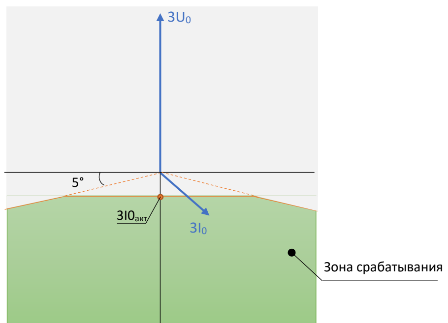
Рисунок 3.16 – Диаграмма срабатывания реле активного тока нулевой последовательности
