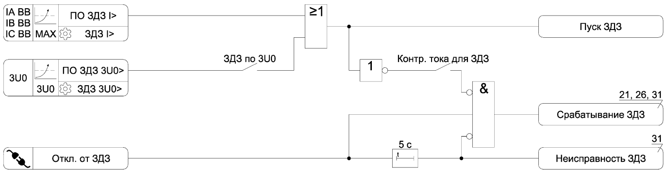
Рисунок А.3 – Функциональная схема алгоритма ЗДЗ
