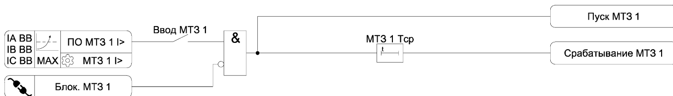
Рисунок 3.4 – Функциональная схема алгоритма МТЗ
