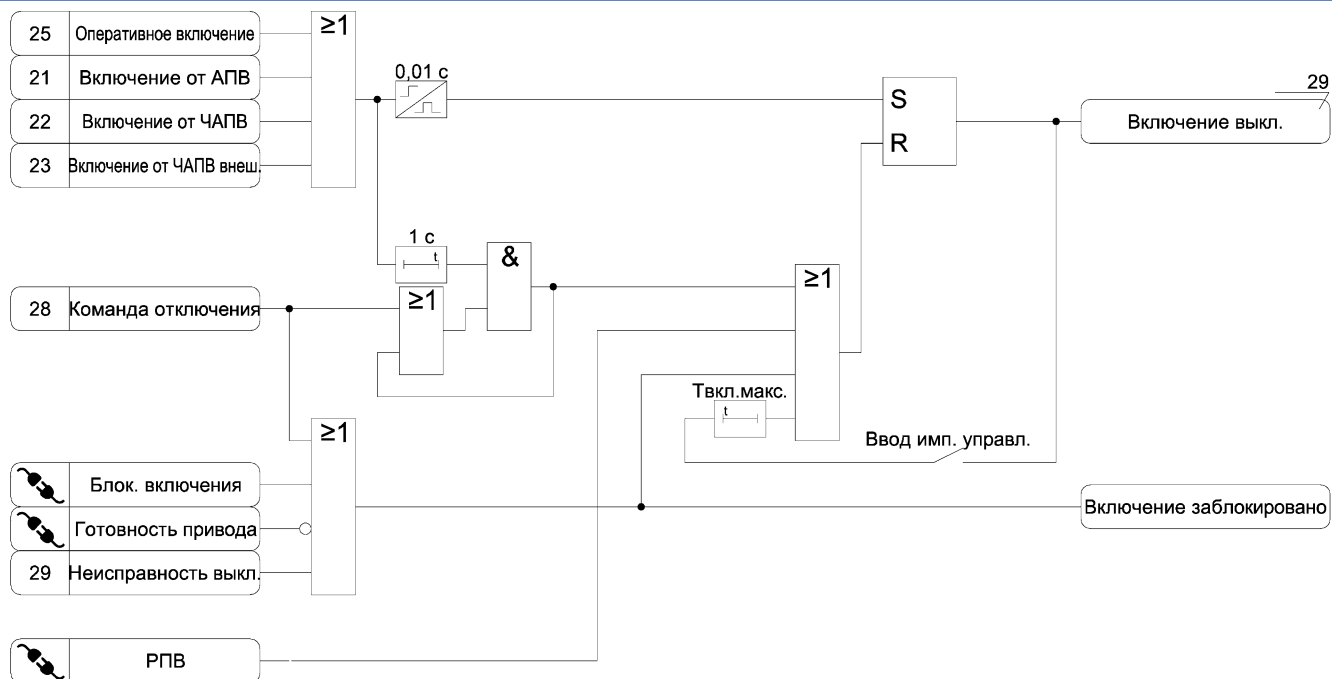
Рисунок А.27 – Функциональная схема алгоритма включения выключателя
