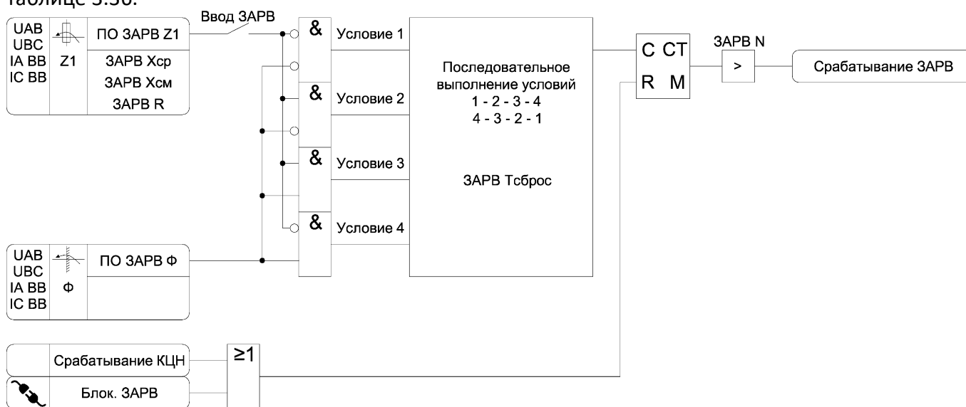
Рисунок 3.23 – Функциональная схема алгоритма ЗАРВ
