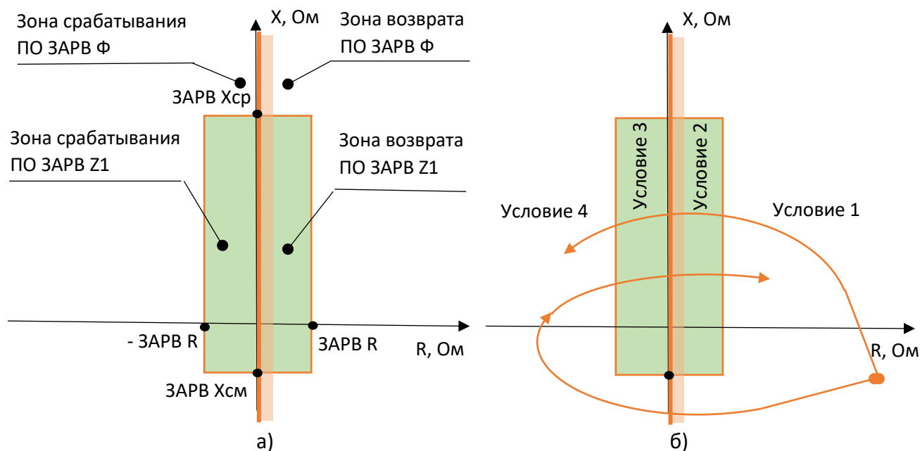
Рисунок 3.24 Характеристика срабатывания ЗАРВ (а) и годограф сопротивления при асинхронном ходе (б)
