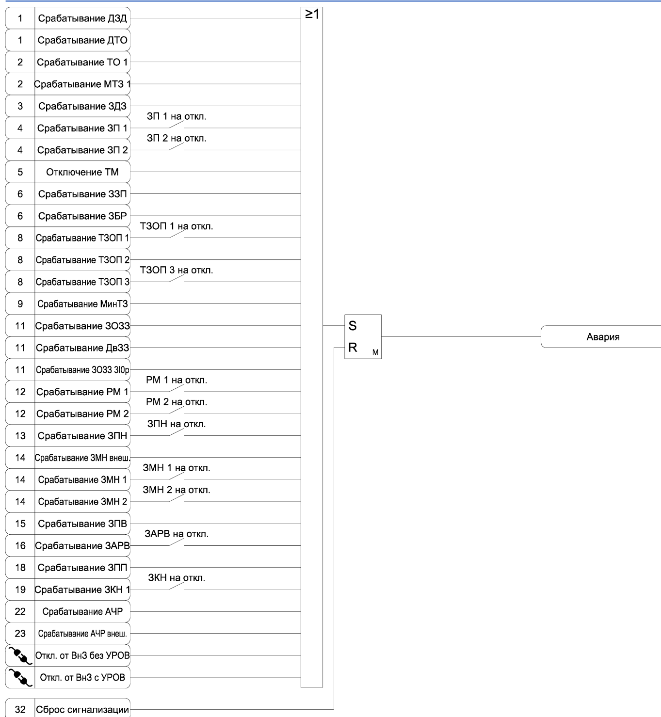
Рисунок А.31 б) – Функциональная схема алгоритма сигнализации
