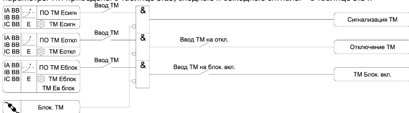
Рисунок 3.8 – Функциональная схема алгоритма ТМ
