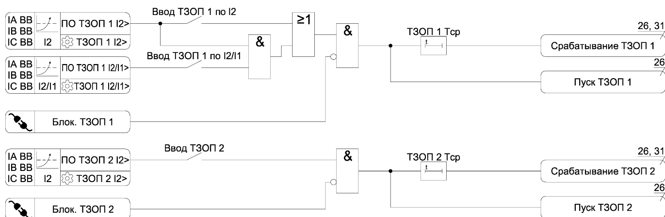
Рисунок А.8 а) – Функциональная схема алгоритма ТЗОП
