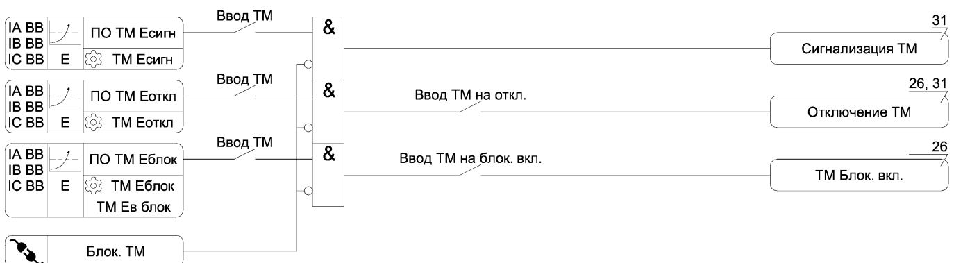
Рисунок А.5 – Функциональная схема алгоритма ТМ
