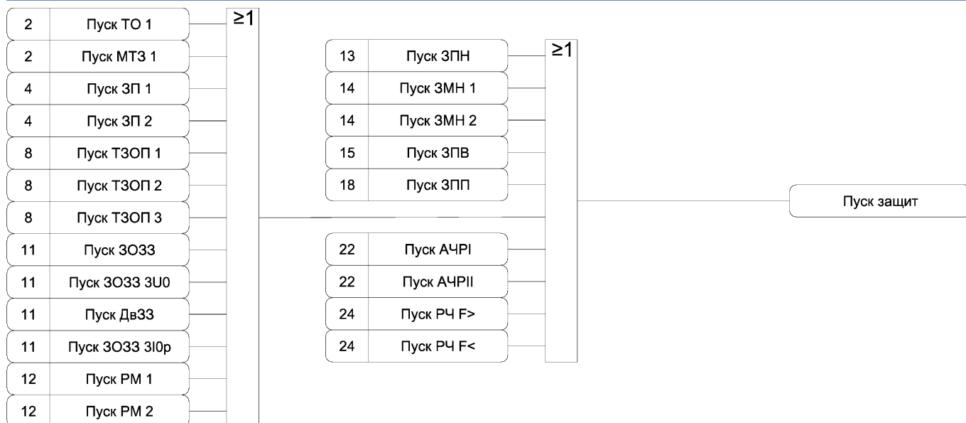
Рисунок А.26 а)– Функциональная схема алгоритма состояния защит
