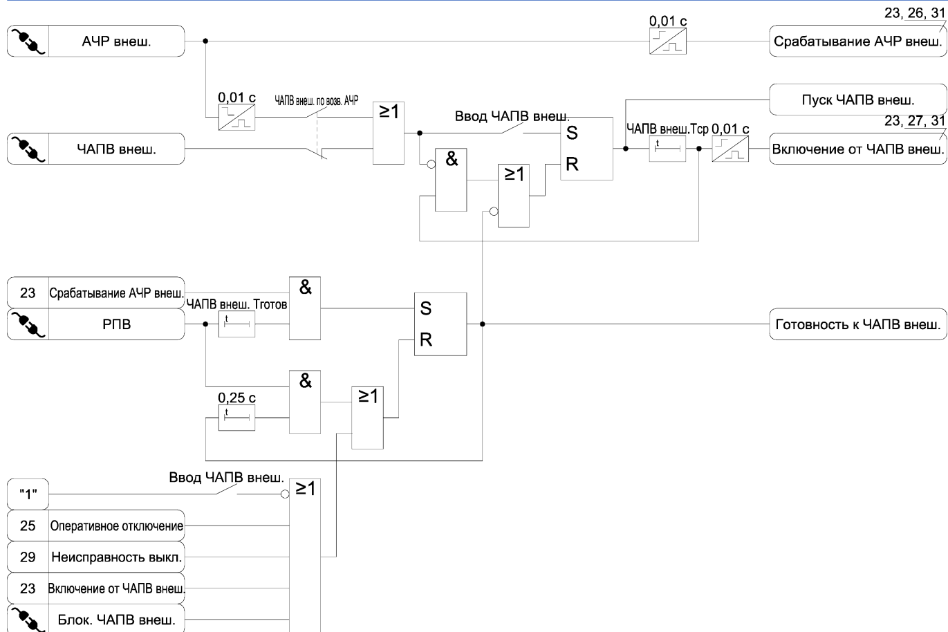
Рисунок А.23 – Функциональная схема алгоритма АЧР и ЧАПВ от внешнего устройства
