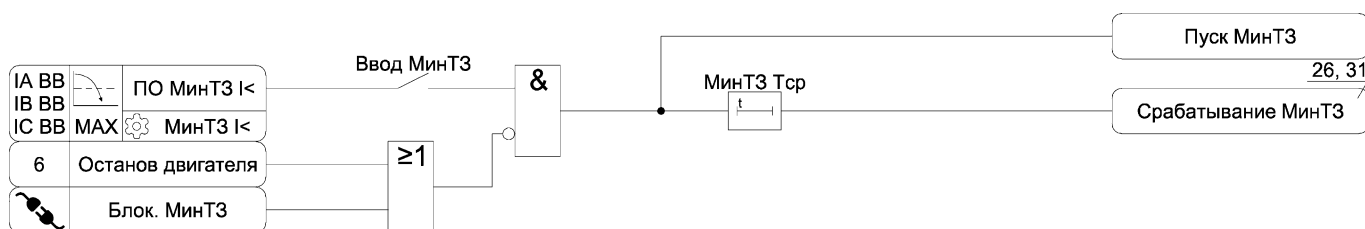
Рисунок А.9 – Функциональная схема алгоритма МинТЗ
