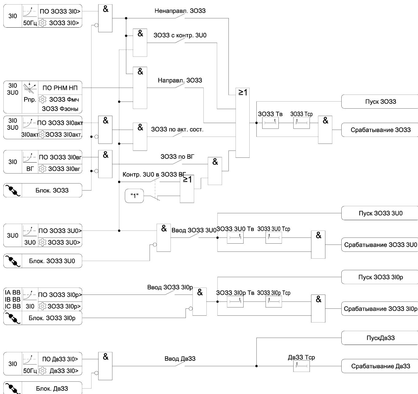
Рисунок 3.14 – Функциональная схема алгоритма ЗОЗЗ
