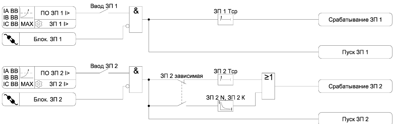
Рисунок 3.7 – Функциональная схема алгоритма ЗП
