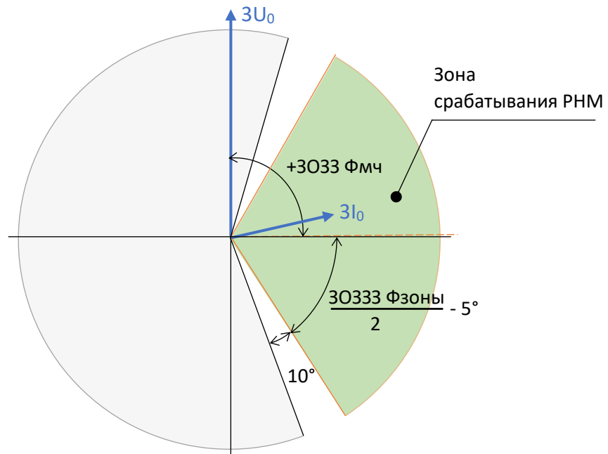
Рисунок 3.15 – Диаграмма срабатывания реле направления мощности нулевой последовательности
