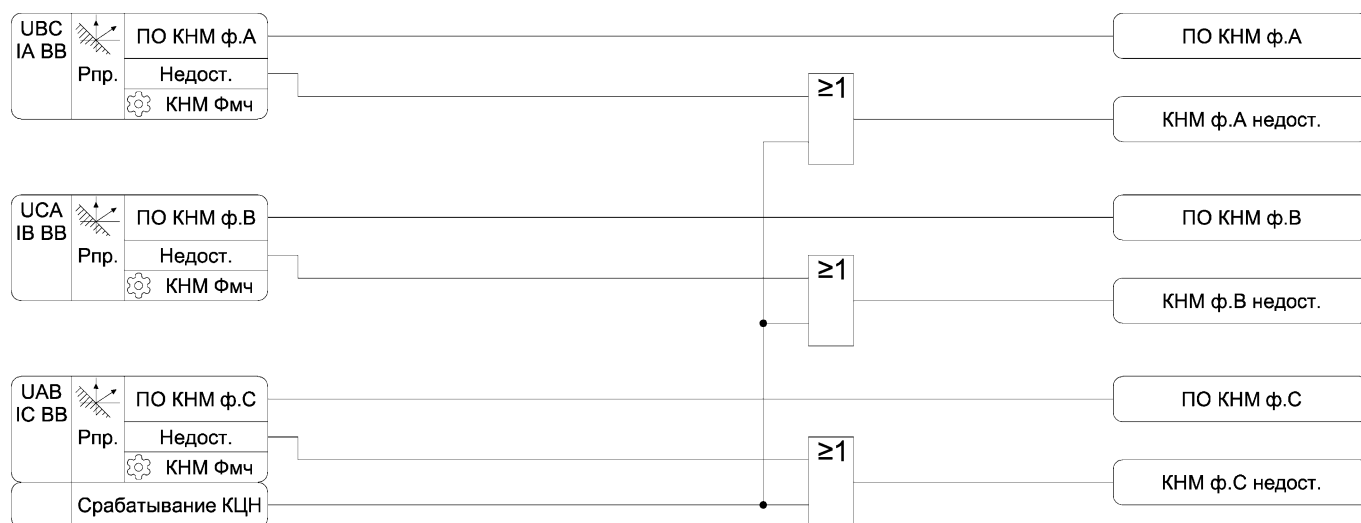
Рисунок 3.25 – Функциональная схема алгоритма КНМ
