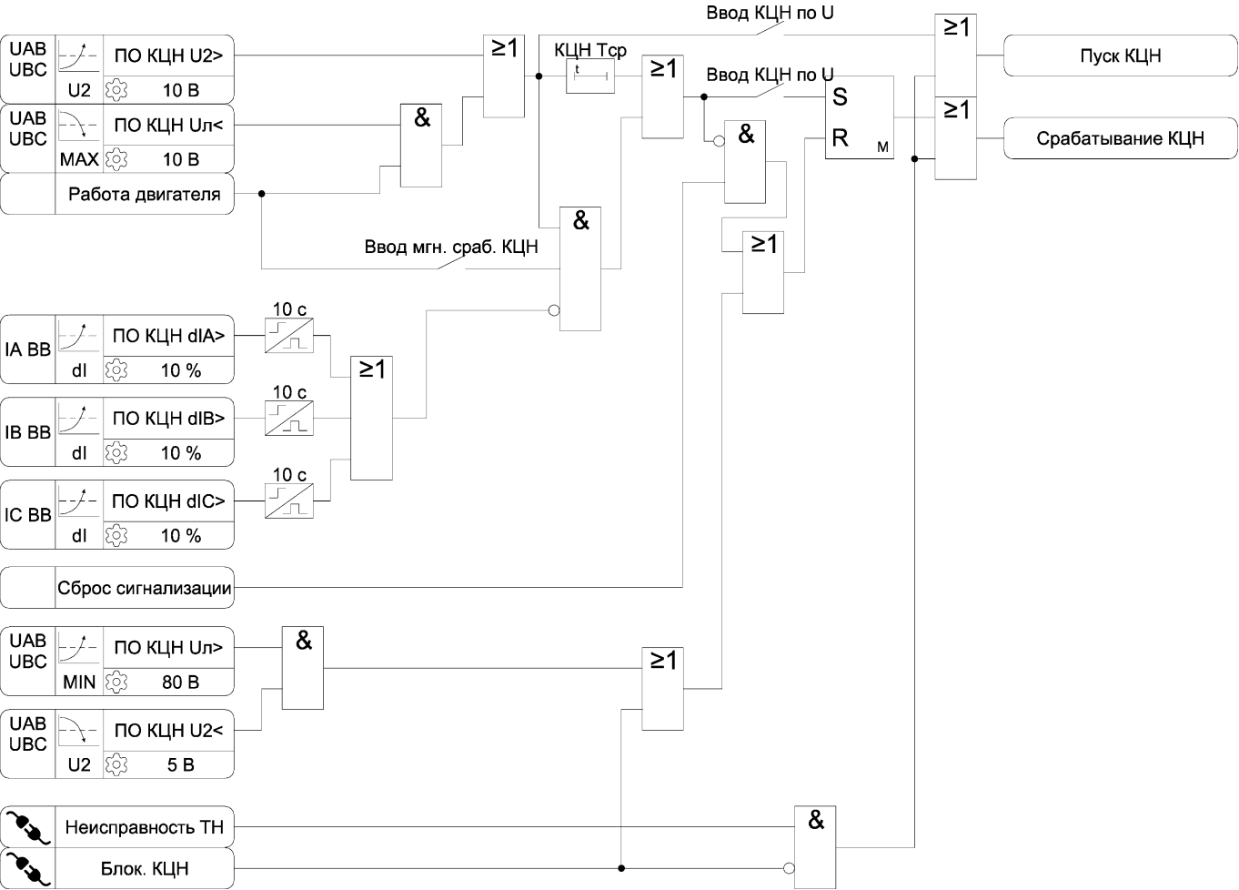
Рисунок 3.40 – Функциональная схема алгоритма КЦН
