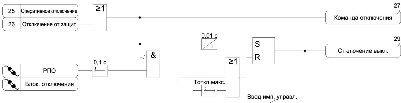
Рисунок А.28 – Функциональная схема алгоритма отключения выключателя
