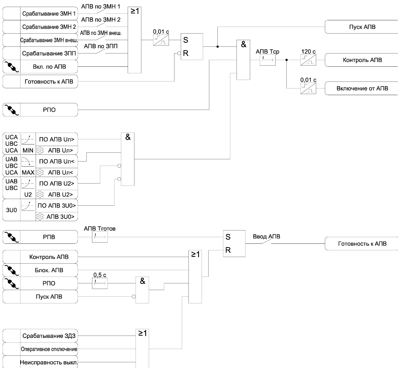
Рисунок 3.31 – Функциональная схема алгоритма АПВ
