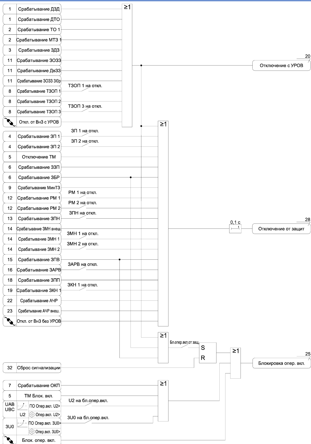
Рисунок А.26 б)– Функциональная схема алгоритма состояния защит
