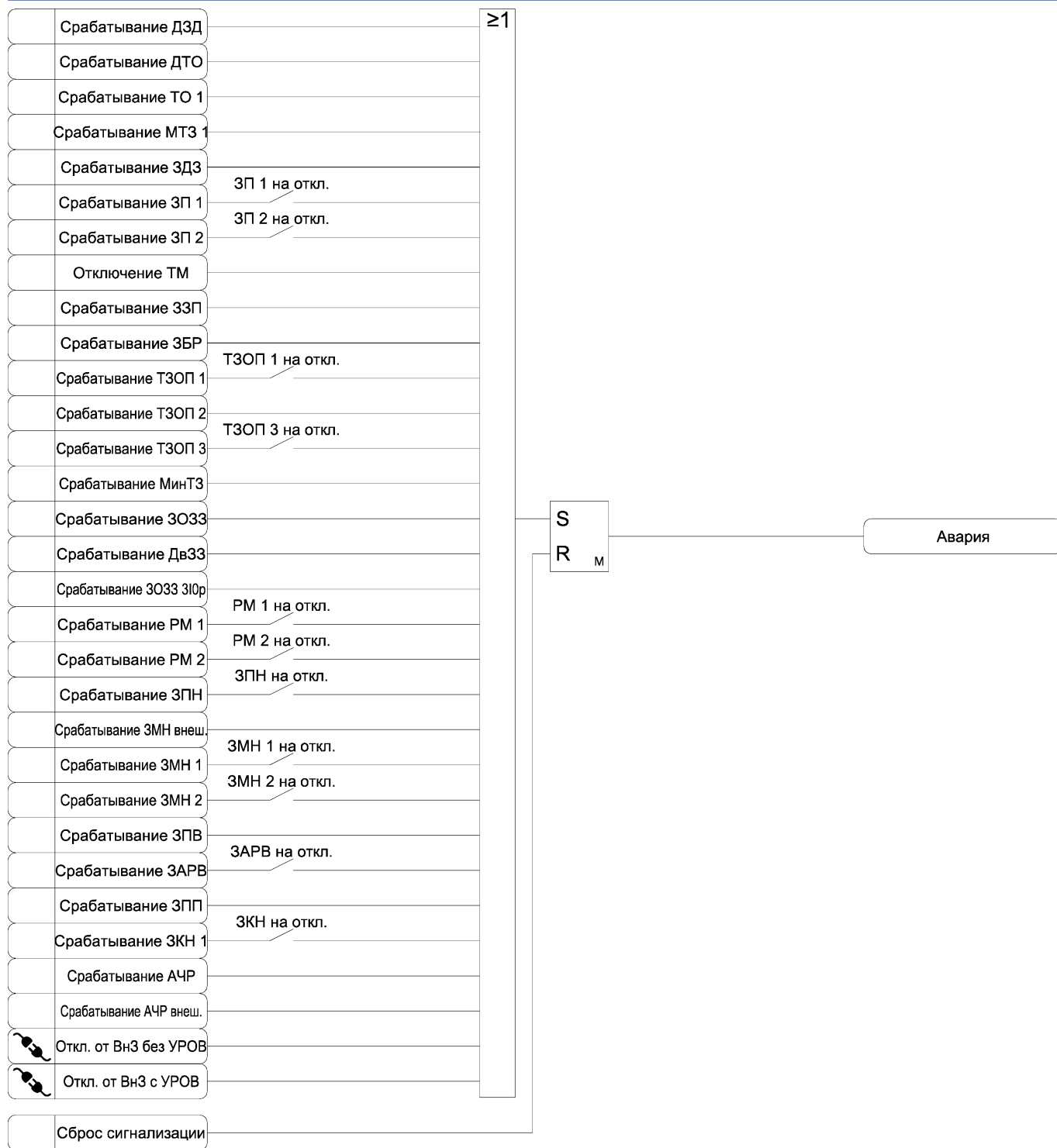
Рисунок 3.41 б) – Функциональная схема алгоритма сигнализации
