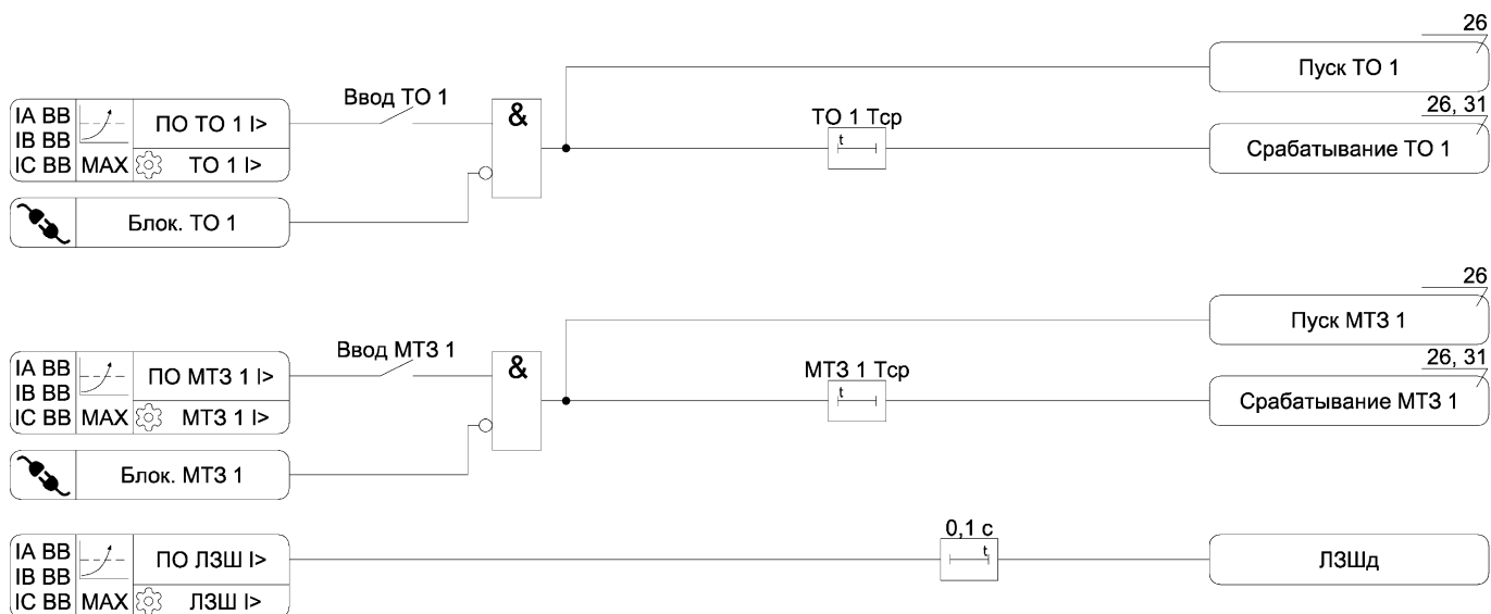
Рисунок А.2 – Функциональная схема алгоритма токовых защит
