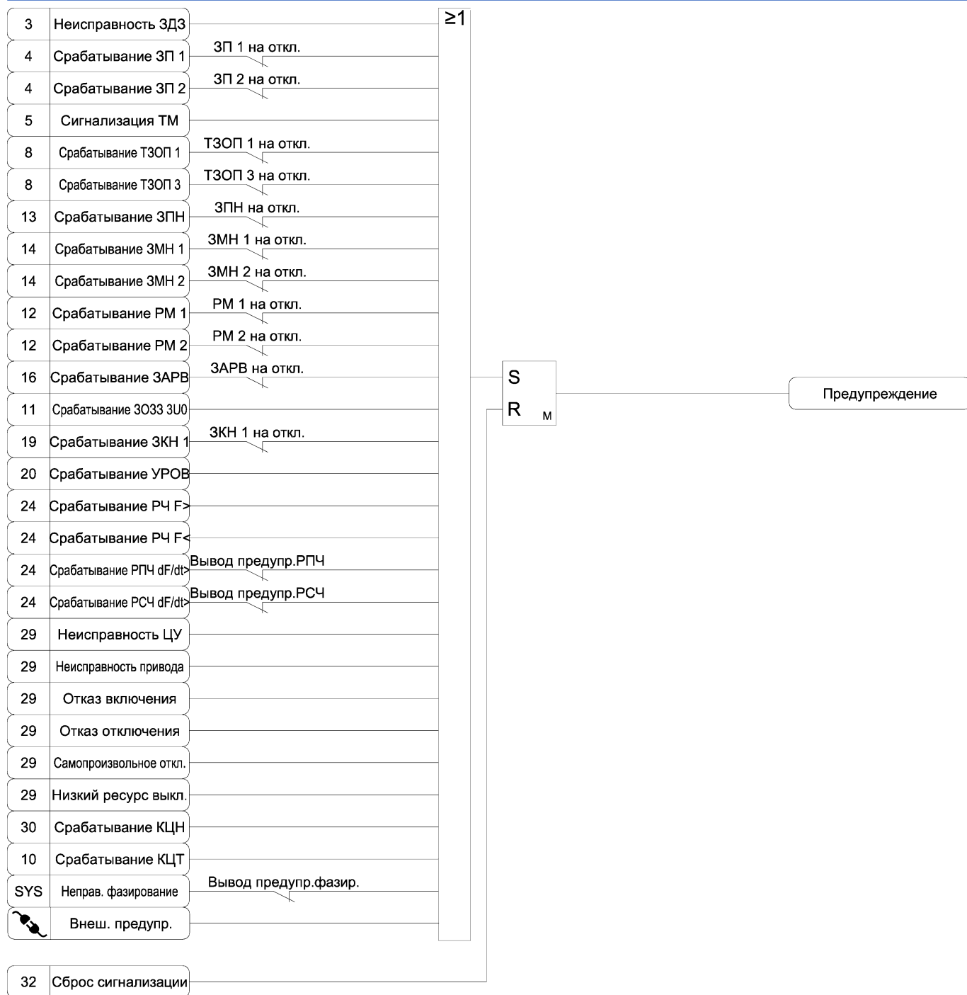
Рисунок А.31 в) – Функциональная схема алгоритма сигнализации
