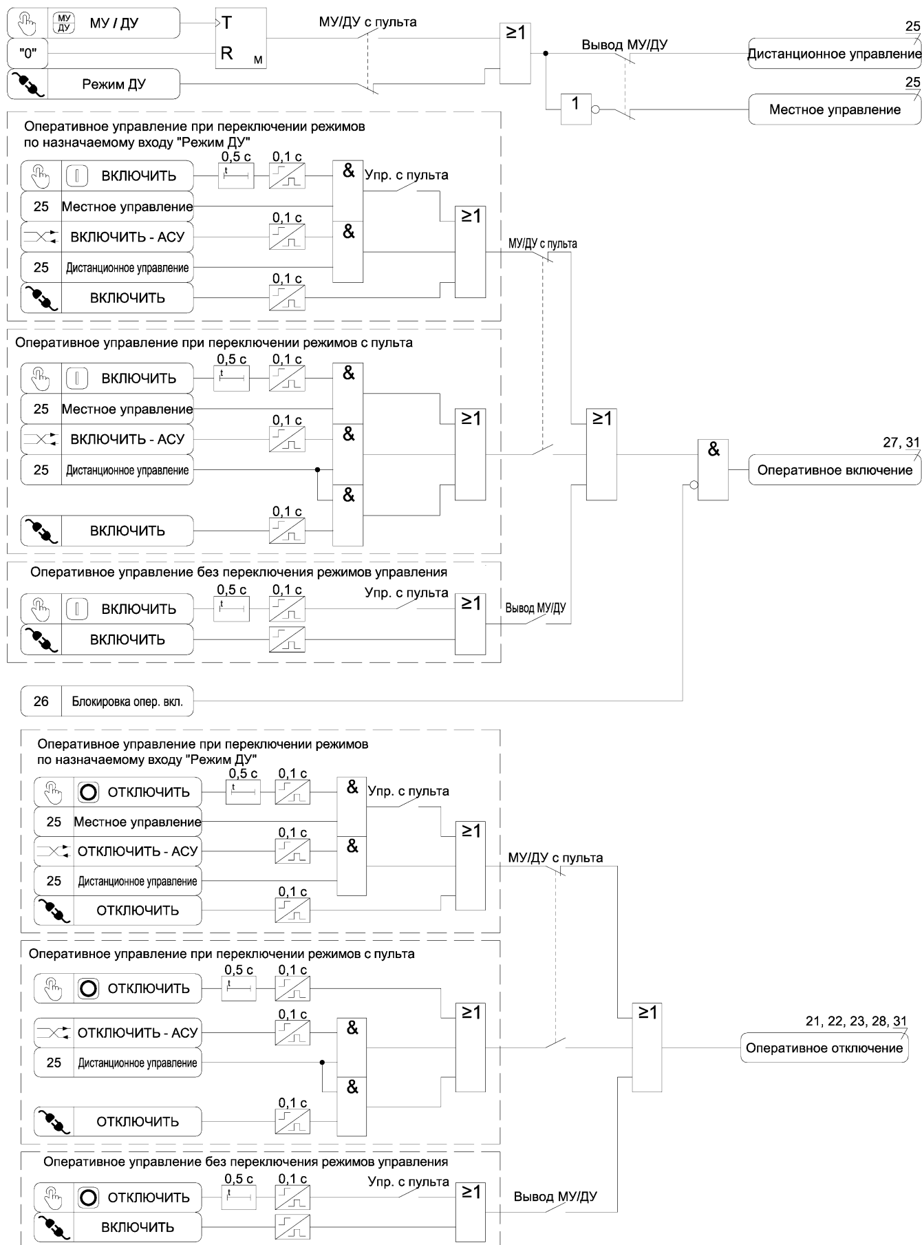
Рисунок А.25 – Функциональная схема алгоритма оперативного управления выключателем
