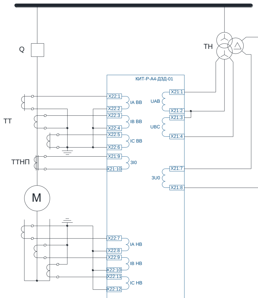
Рисунок 1.1 – Варианты подключения устройства
