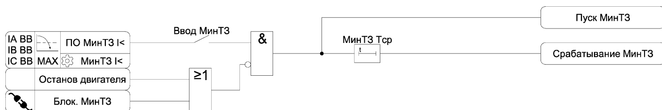
Рисунок 3.12 – Функциональная схема алгоритма МинТЗ
