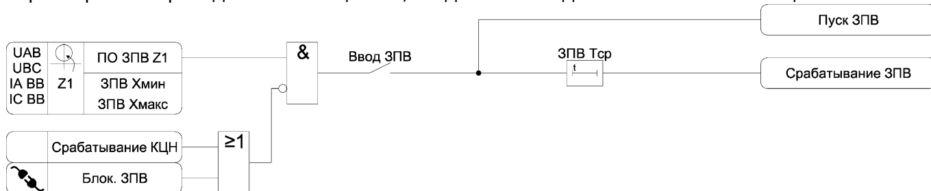
Рисунок 3.21 – Функциональная схема алгоритма ЗПВ
