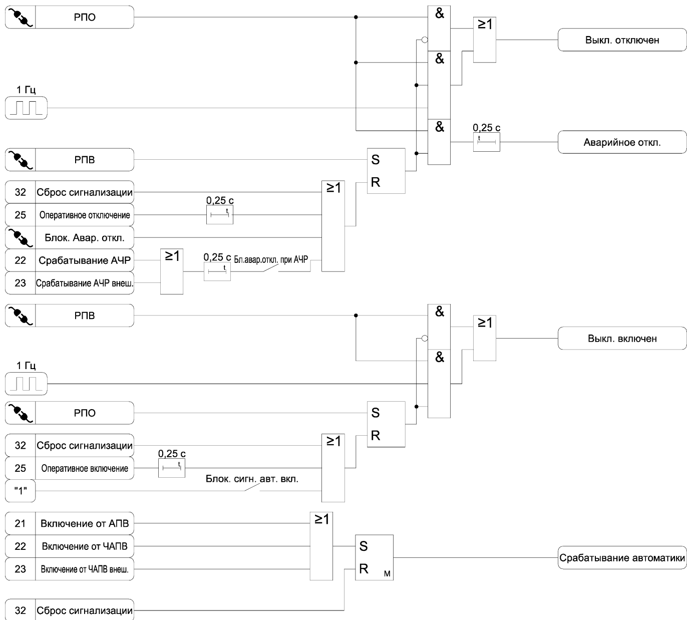
Рисунок А.31 а) – Функциональная схема алгоритма сигнализации
