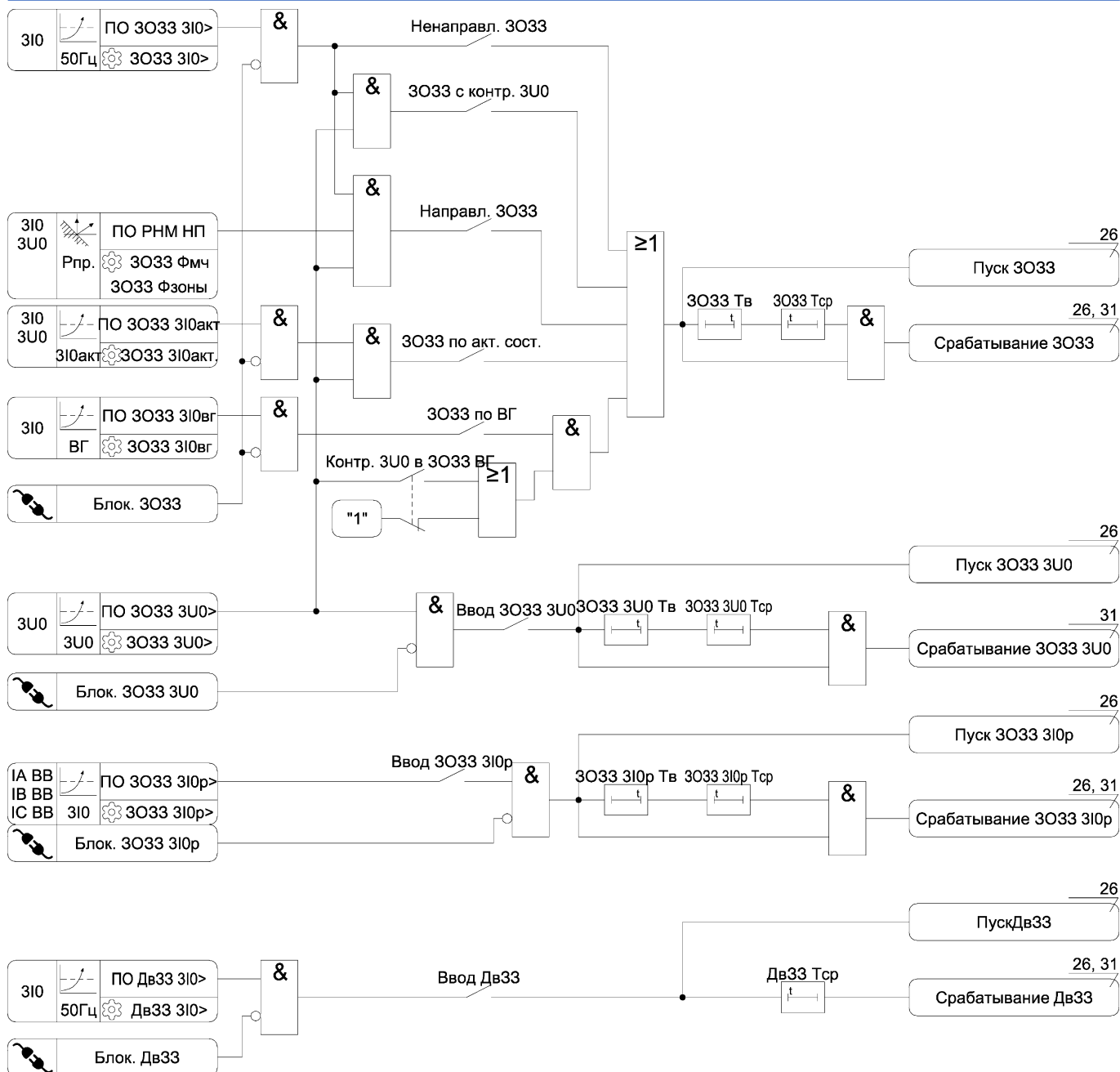
Рисунок А.11 – Функциональная схема алгоритма 3033
