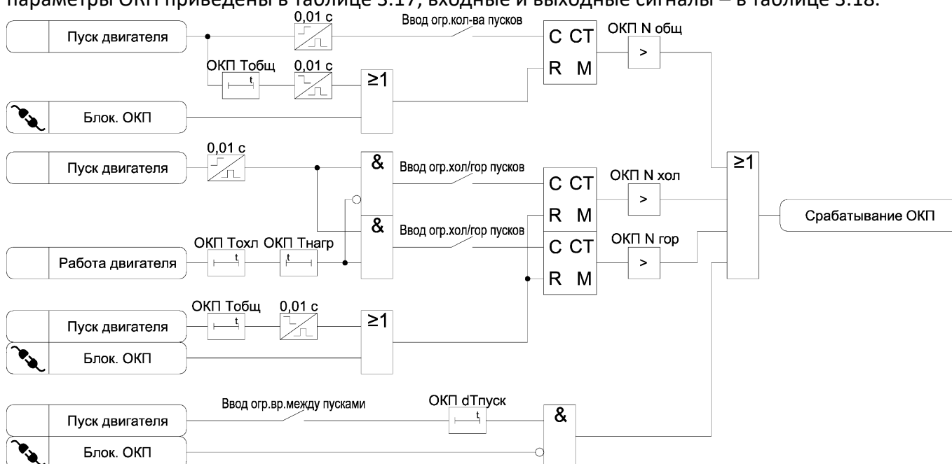
Рисунок 3.10 – Функциональная схема алгоритма ОКП
