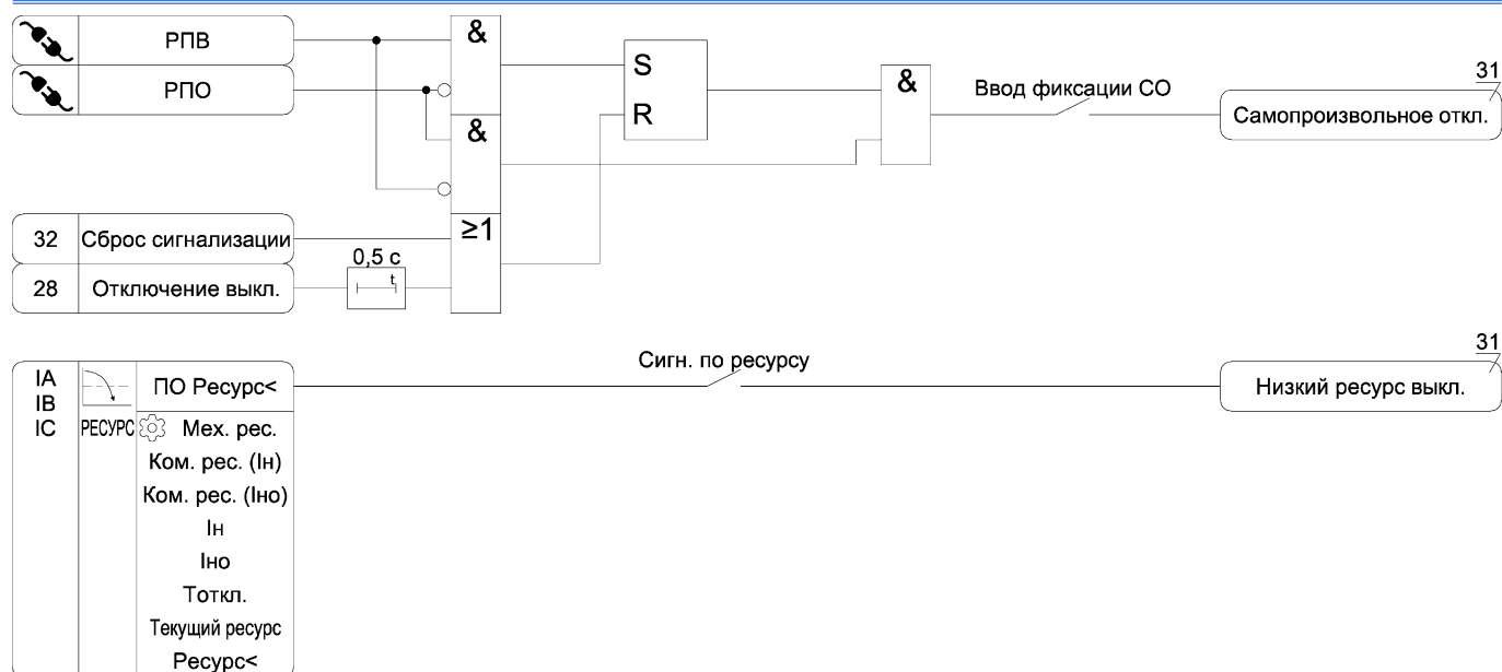
Рисунок А.29 б) – Функциональная схема алгоритма диагностики выключателя
