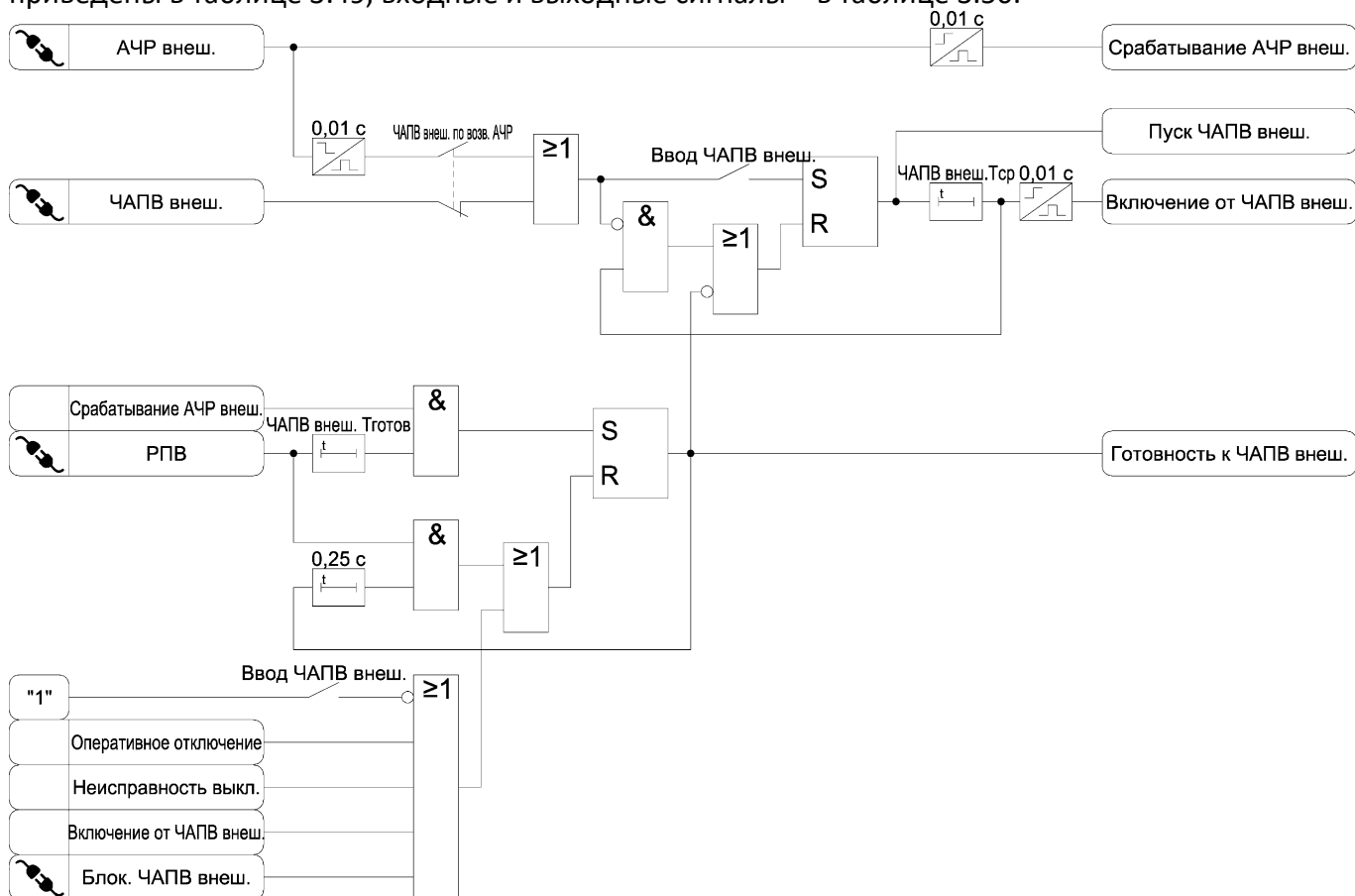
Рисунок 3.33 – Функциональные схемы алгоритмов АЧР и ЧАПВ от внешнего устройства
