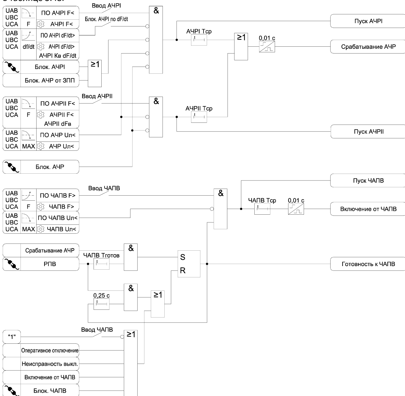
Рисунок 3.32 – Функциональные схемы алгоритмов АЧР и ЧАПВ
