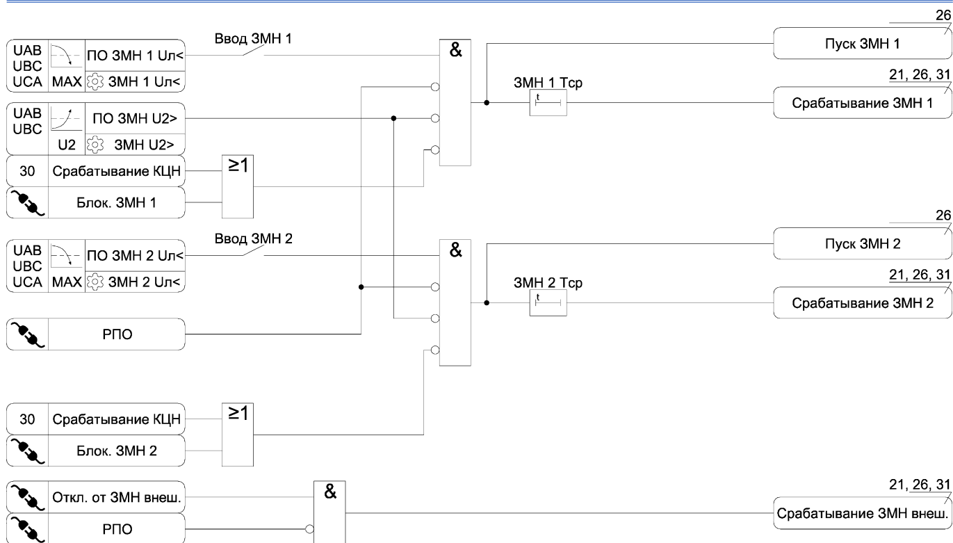
Рисунок А.14 – Функциональная схема алгоритма 3МН
