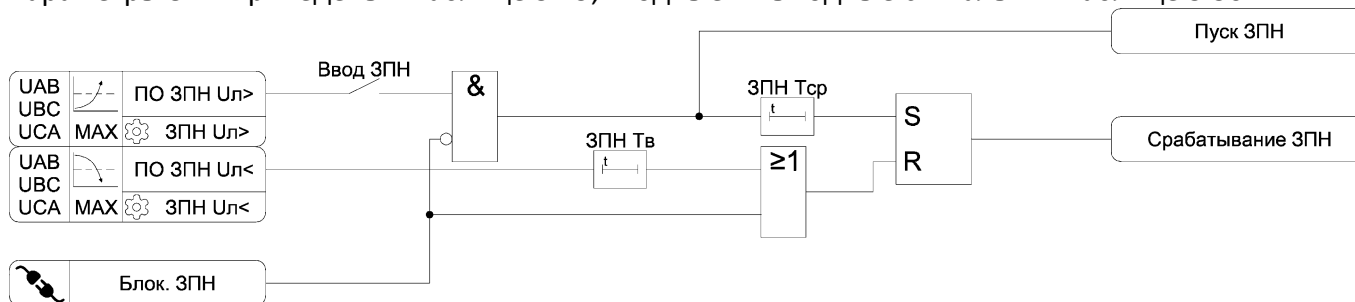
Рисунок 3.19 – Функциональная схема алгоритма ЗПН
