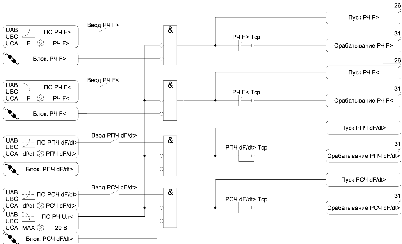
Рисунок А.24 – Функциональная схема алгоритма защиты от повышения и снижения частоты
