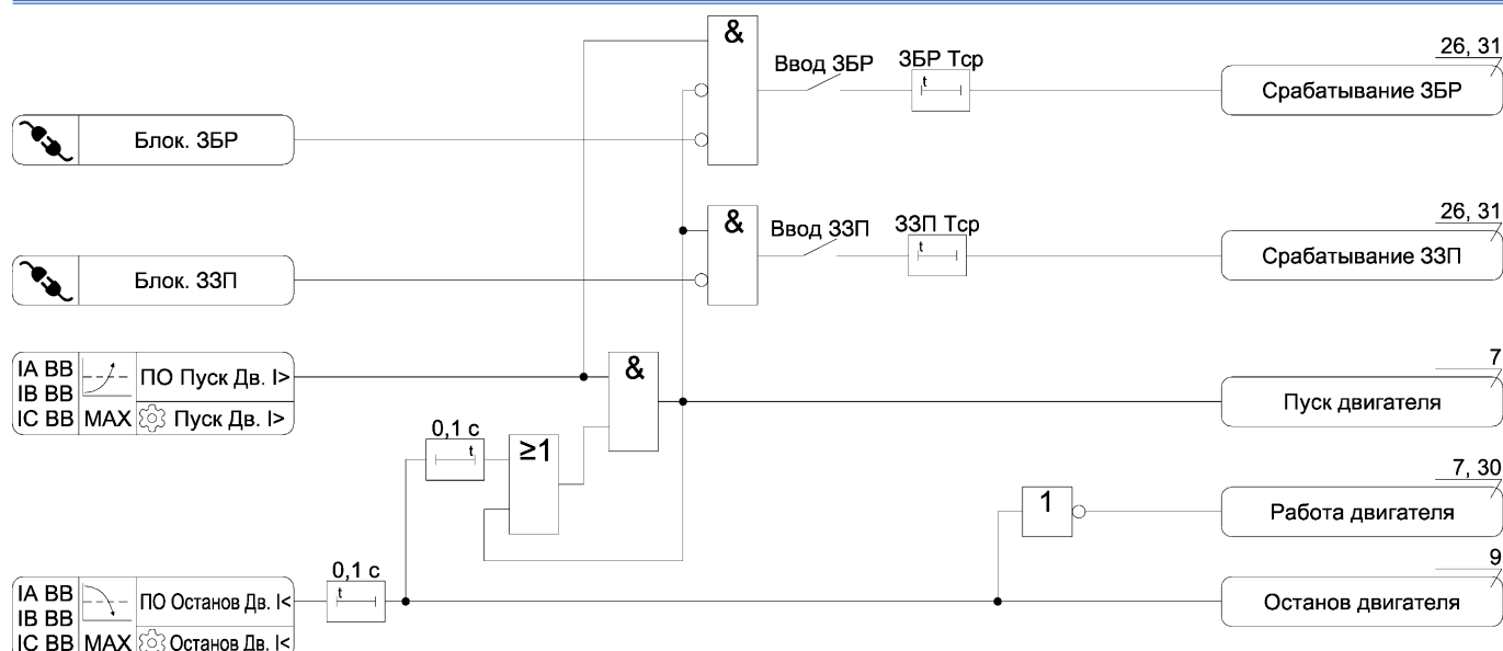
Рисунок А.6 – Функциональная схема алгоритма 3ЗП и 3БР
