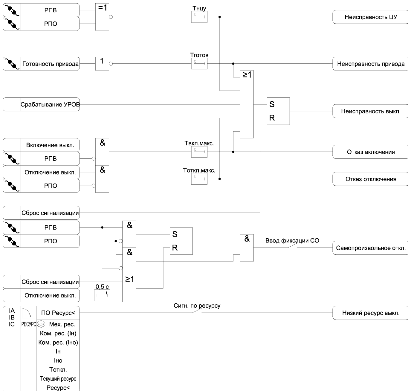
Рисунок 3.39 – Функциональная схема алгоритма диагностики выключателя
