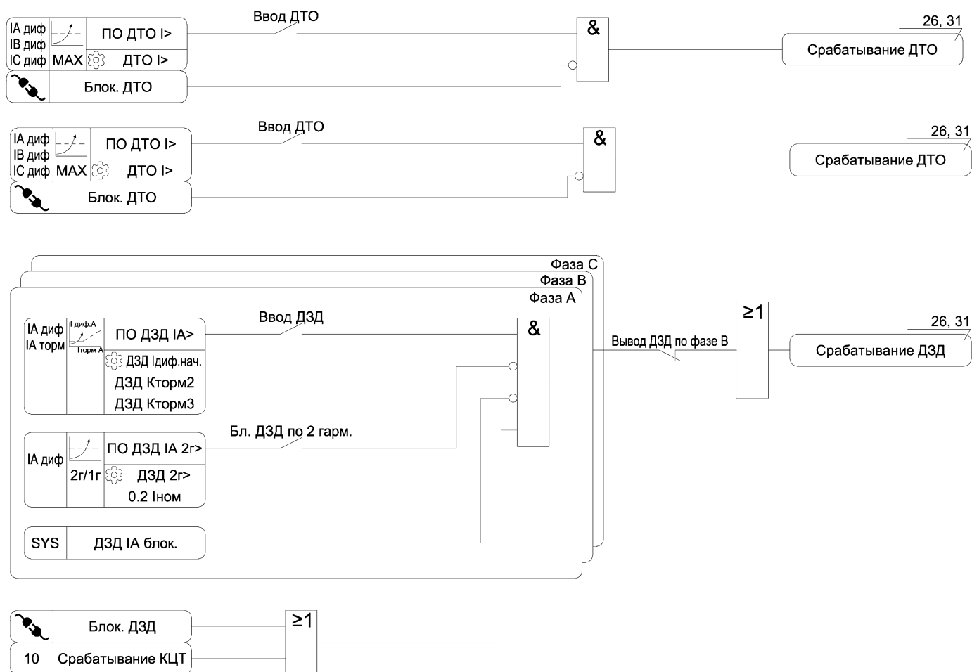
Рисунок А.1 – Функциональная схема алгоритма ДЗД
