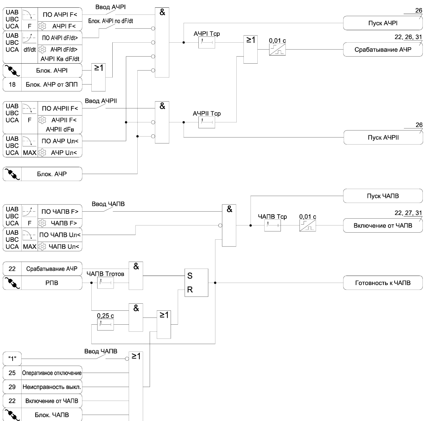
Рисунок А.22 – Функциональная схема алгоритма АЧР и ЧАПВ
