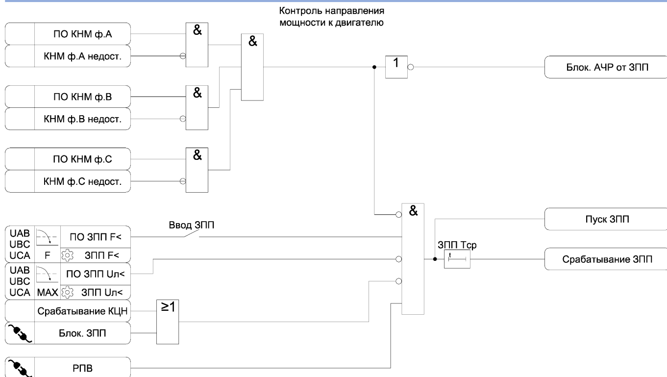
Рисунок 3.27 – Функциональная схема алгоритма ЗПП
