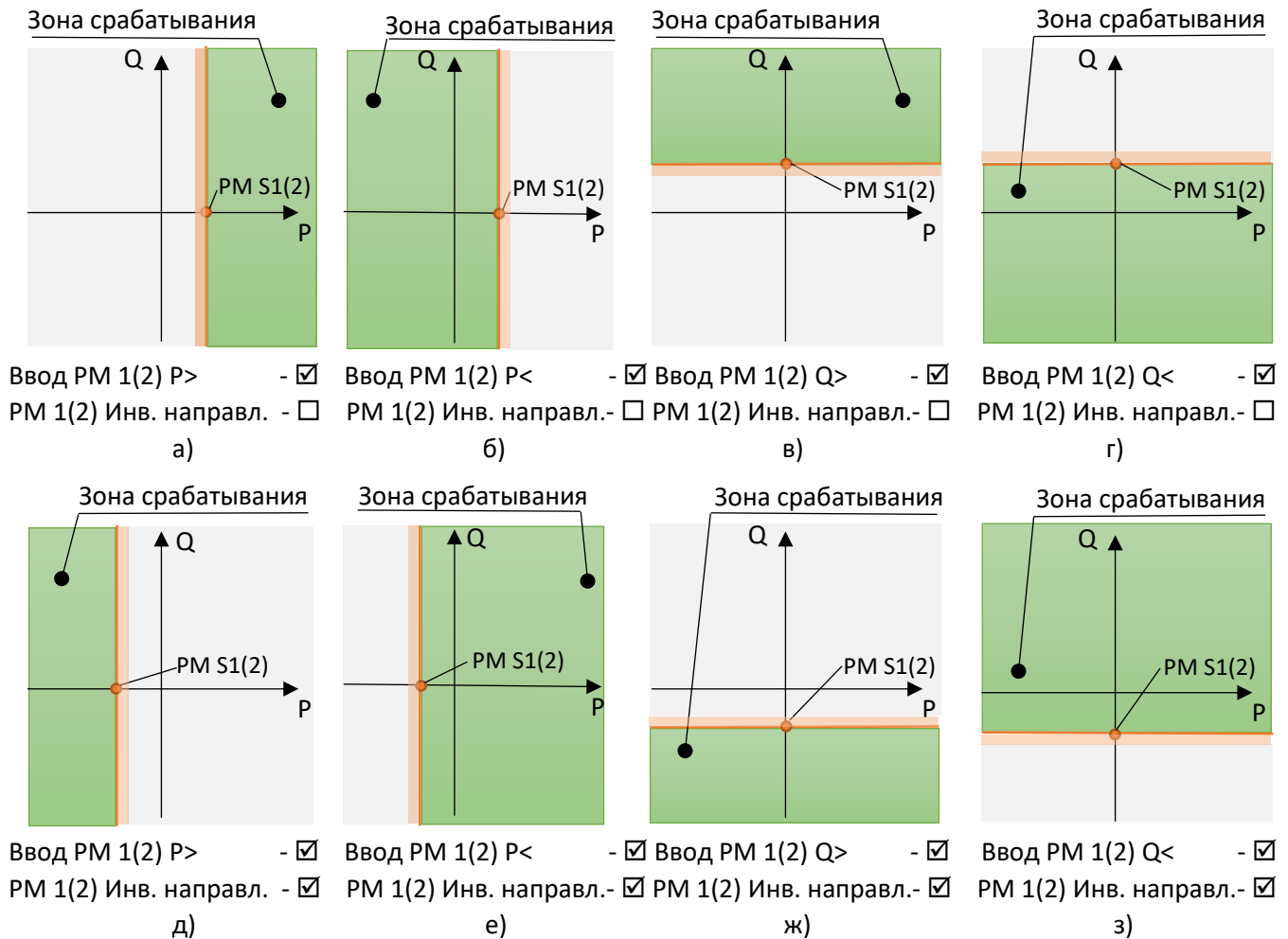
Рисунок 3.18 – Диаграмма срабатывания реле активного тока нулевой последовательности
