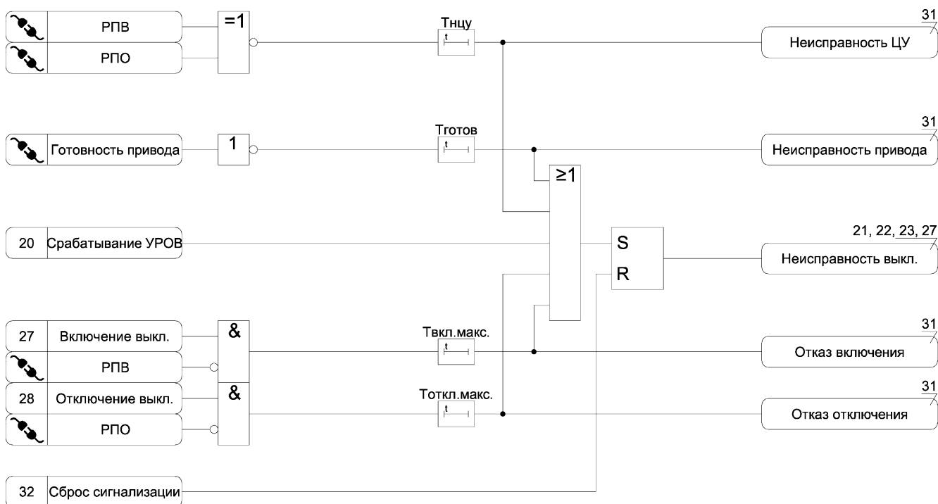
Рисунок А.29 а) – Функциональная схема алгоритма диагностики выключателя
