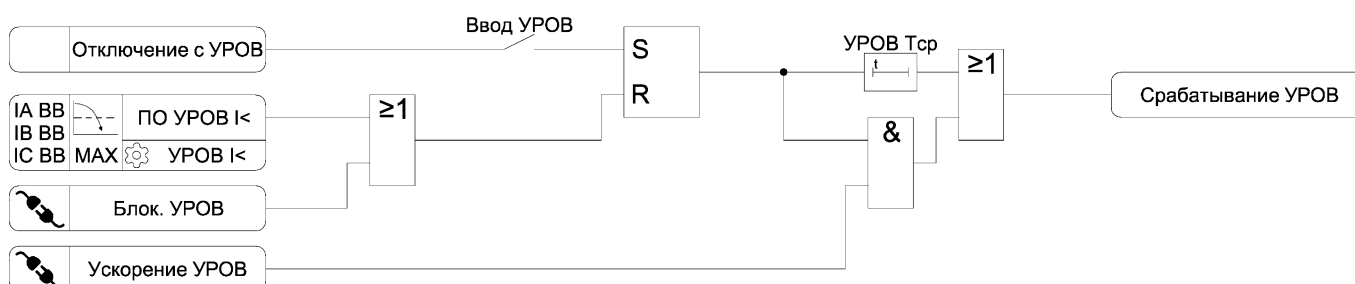
Рисунок 3.30 – Функциональная схема алгоритма УРОВ
