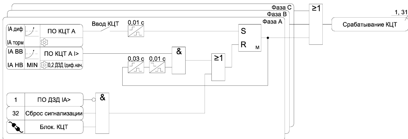
Рисунок А.10 – Функциональная схема алгоритма КЦТ
