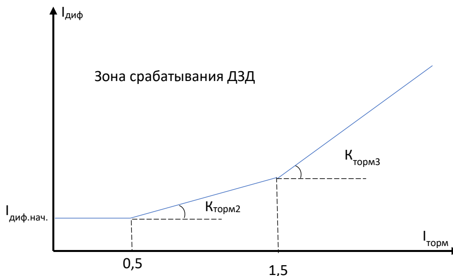
Рисунок 3.2 – Характеристика срабатывания ДЗД
