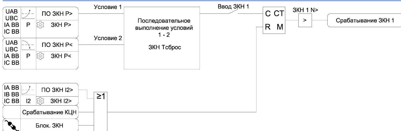
Рисунок 3.28 – Функциональная схема алгоритма ЗКН
