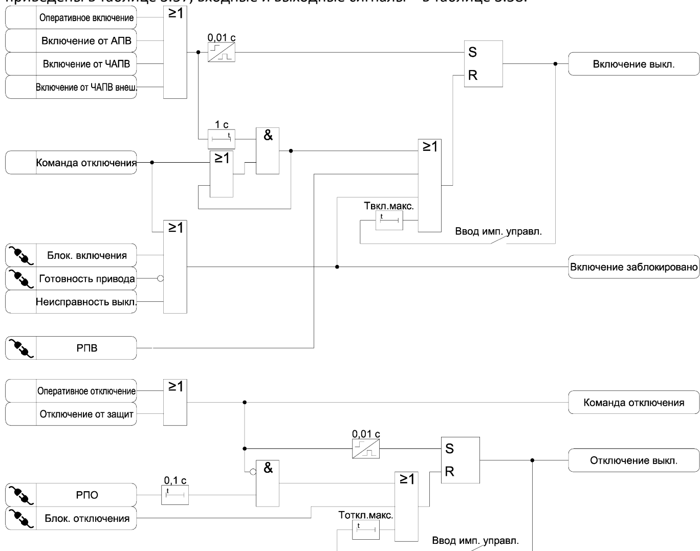
Рисунок 3.38 – Функциональная схема алгоритма управления выключателем
