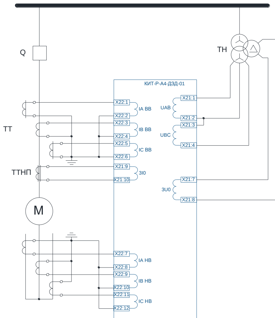
а) схема с тремя ТТ
