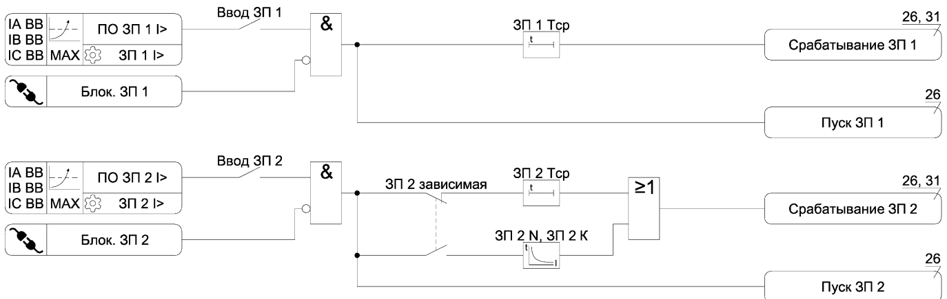
Рисунок А.4 – Функциональная схема алгоритма ЗП
