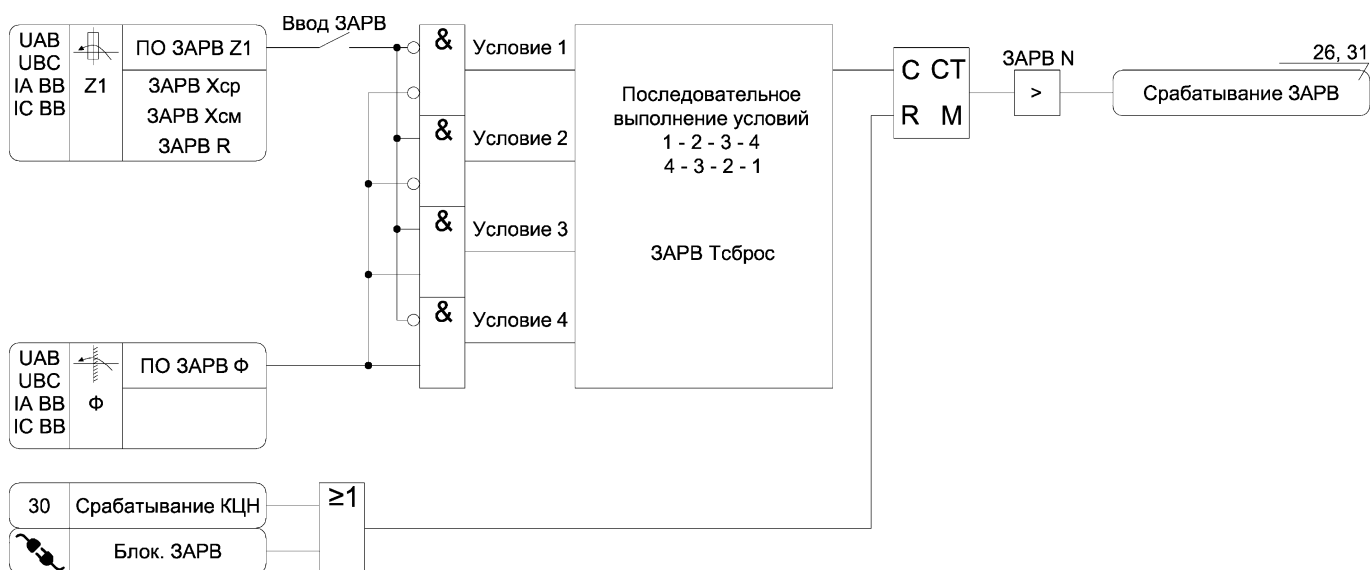
Рисунок А.16 – Функциональная схема алгоритма 3АРВ
