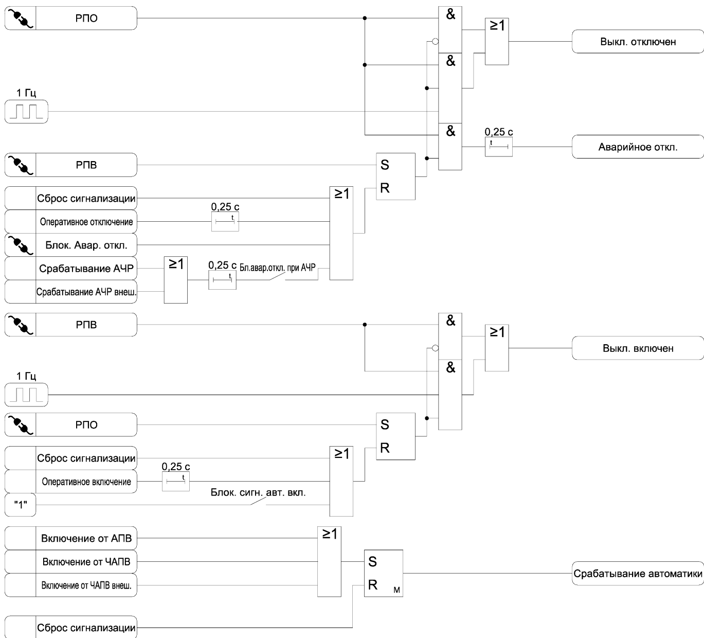
Рисунок 3.41 а) – Функциональная схема алгоритма сигнализации
