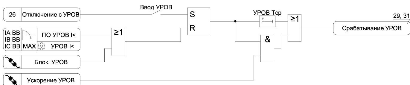
Рисунок А.20 – Функциональная схема алгоритма УРОВ
