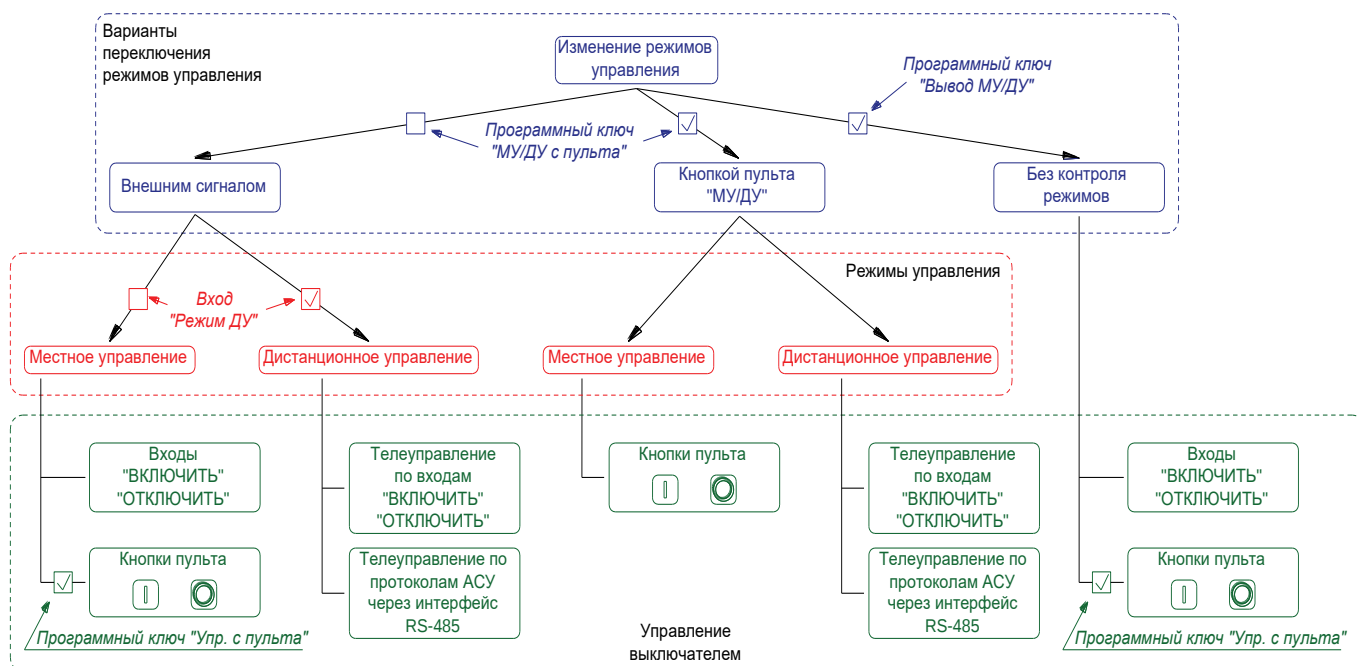
Рисунок 3.36 – Выбор режимов управления
