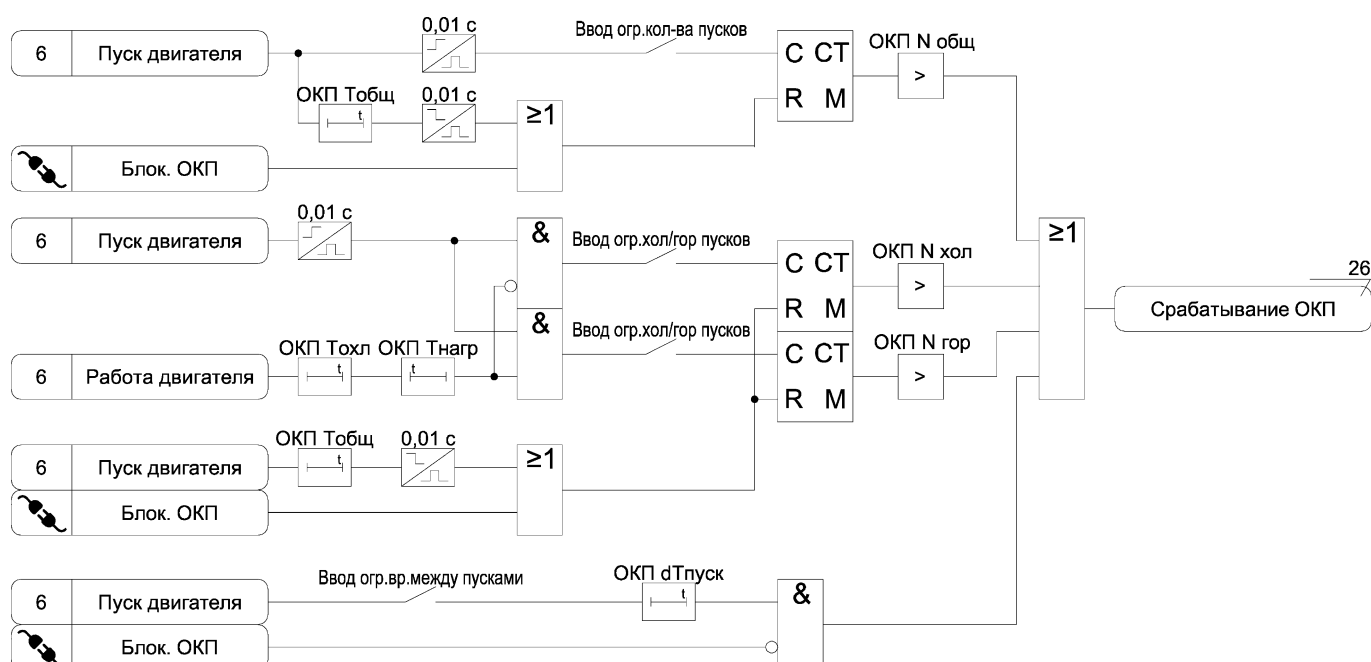
Рисунок А.7 – Функциональная схема алгоритма ОКП
